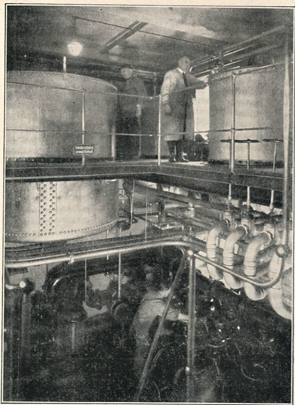
Pump- och ventilanläggning. Kapac. över 300 ton i timmen. Med ca. 200 ventiler fördelas oljan till fabriken's olika avdel.
