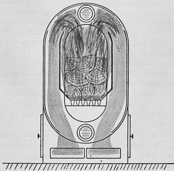
Kuva 2. Arinapeitoksen järjestely halkolämmityksessä (poikkileikkauskuva).
