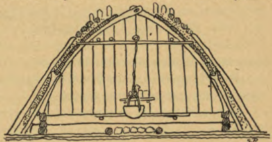
Turvekodan poikkileikkaus: peräpuoli.
