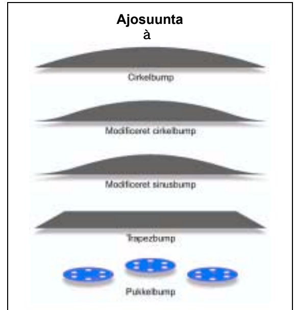
Kuva 3.3 Töyssyjen pituusprofileja. Suomalaiset töyssyt ovat pääosin trapetsimuotoisia. /13/
