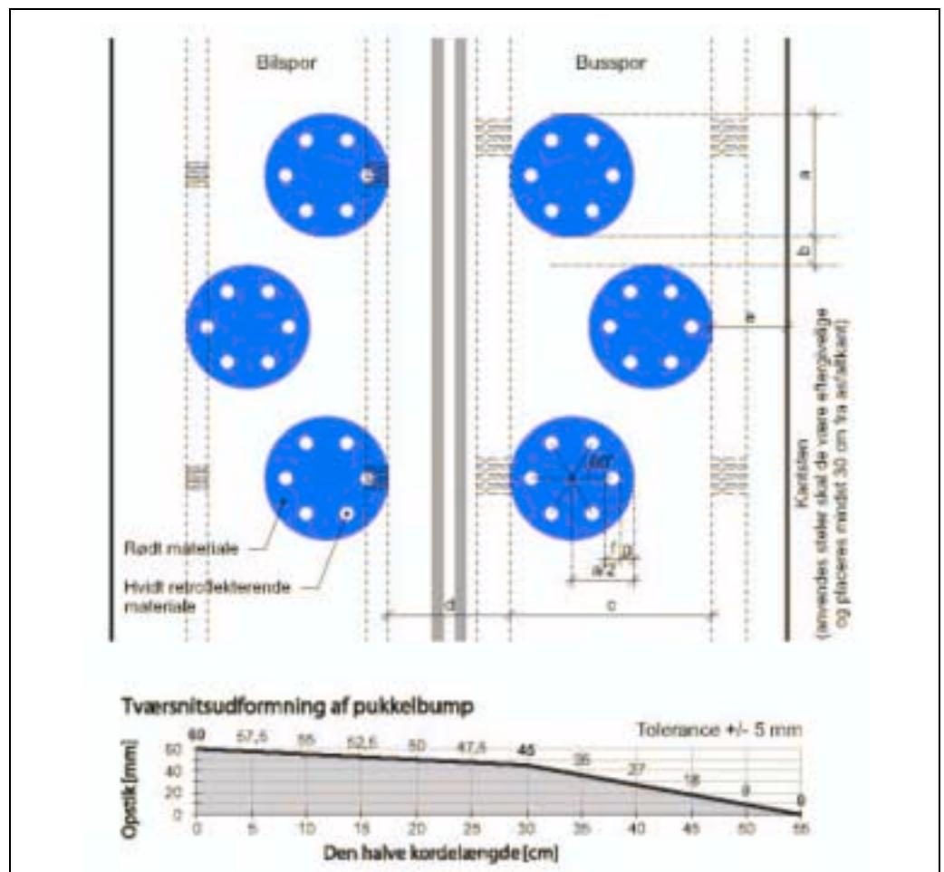
Kuva 3.4 Esimerkki muhkuramallisesta hidasteesta, joka soveltuu erityisesti joukko- liikenteen reiteille. /13/
