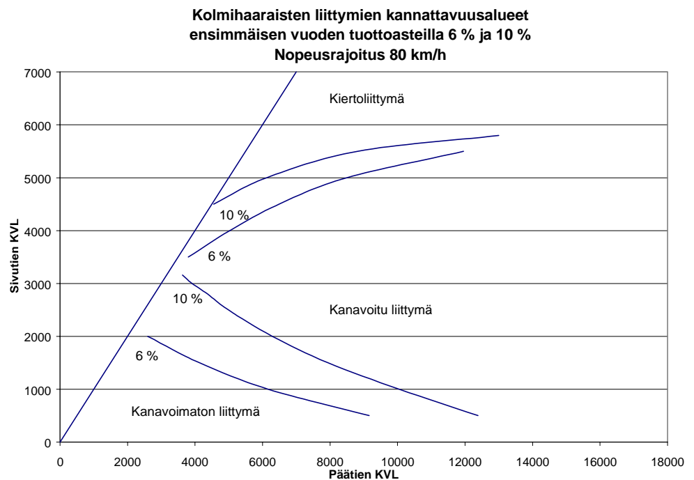
Kuva 4. Kolmihaaraisen liittymien kannattavuusalueet nopeusrajoituksella 80 km/h. Liite 2.
