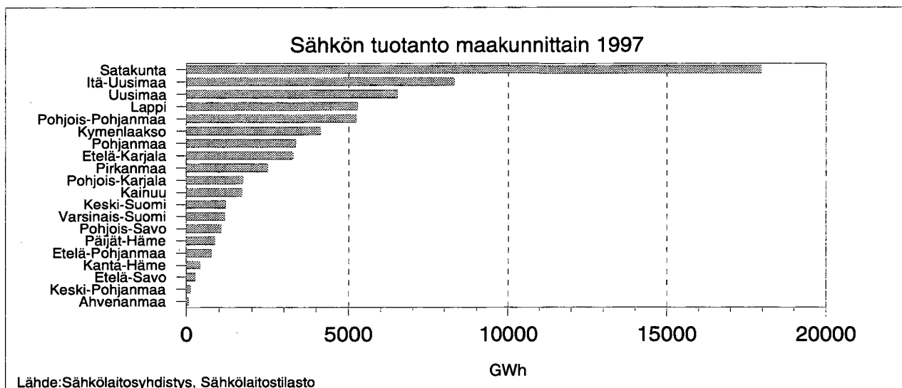
Kuva 176. Sähkön tuotanto maakunnittain 1997.
