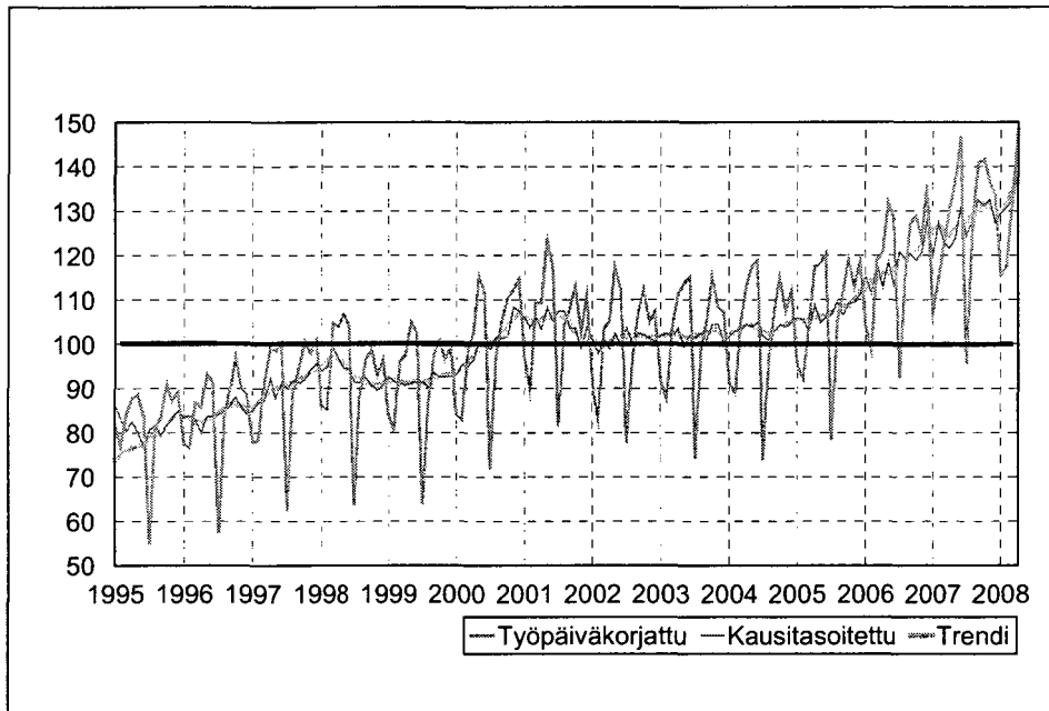
Kuvio 9. Muu metalliteollisuus TOL met - DL, teollisuustuotannon volyymi-indeksi 1995 – 2008 huhtikuu, 2000=100
