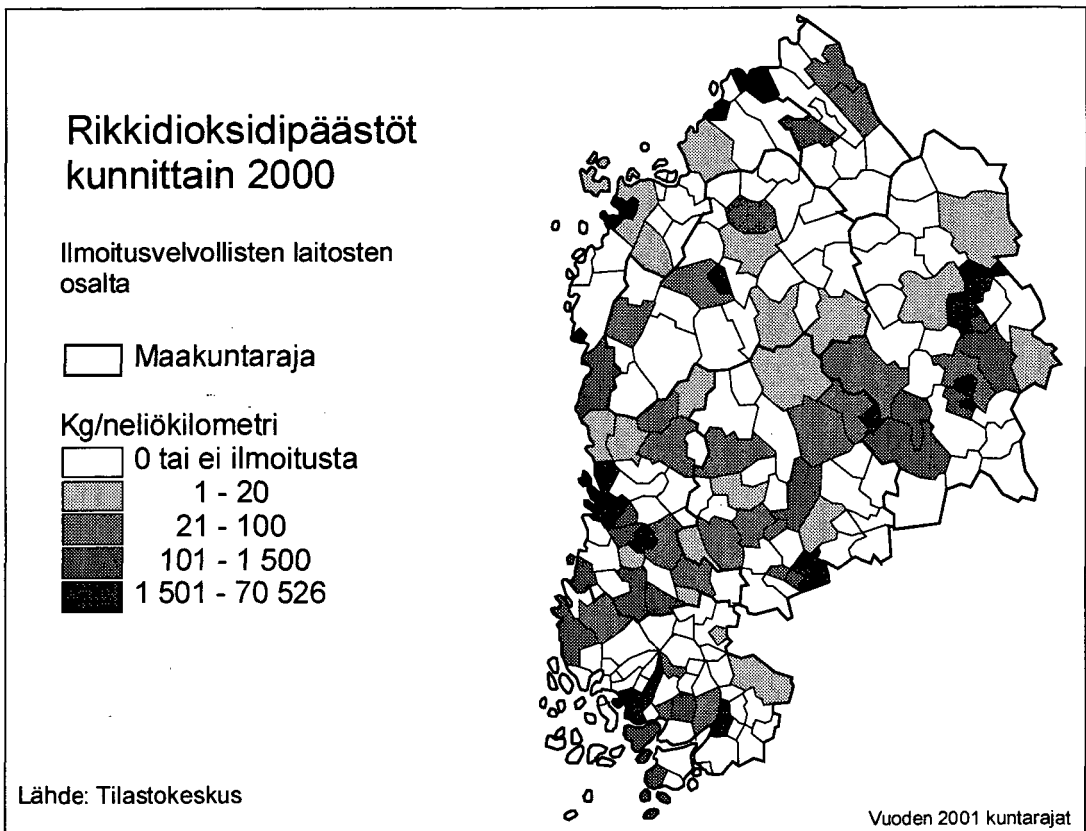
Kuva 135. Rikkidioksidipäästöt ( \text{SO}_2 ) kunnittain 2000.
