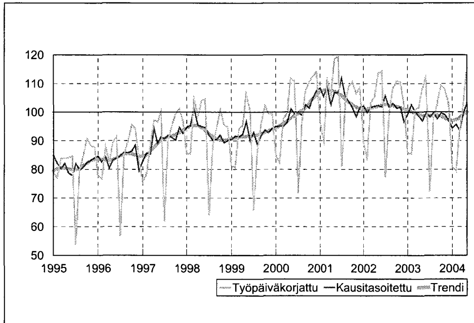
Kuvio 9. Muu metalliteollisuus TOL met - DL, teollisuustuotannon volyymi-indeksi 1995 – 2004 toukokuu, 2000=100
