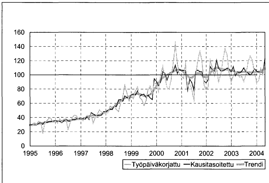
Kuvio 10. Elektroniikka- ja sähkötuotteiden valmistus TOL DL, teollisuustuotannon volyymi-indeksi 1995 – 2004 toukokuu, 2000=100
