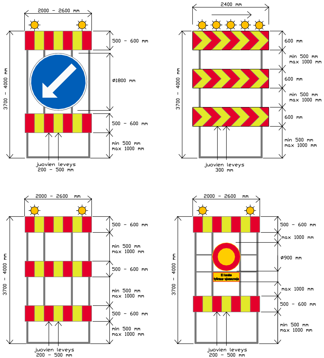
Kuva 2. S3-toimintaympäristöluokan sulkuaidan mitoitus.
