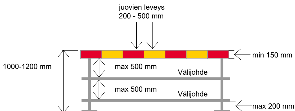
Kuva 9. Esimerkki sulkupuomin mitoituksesta.
