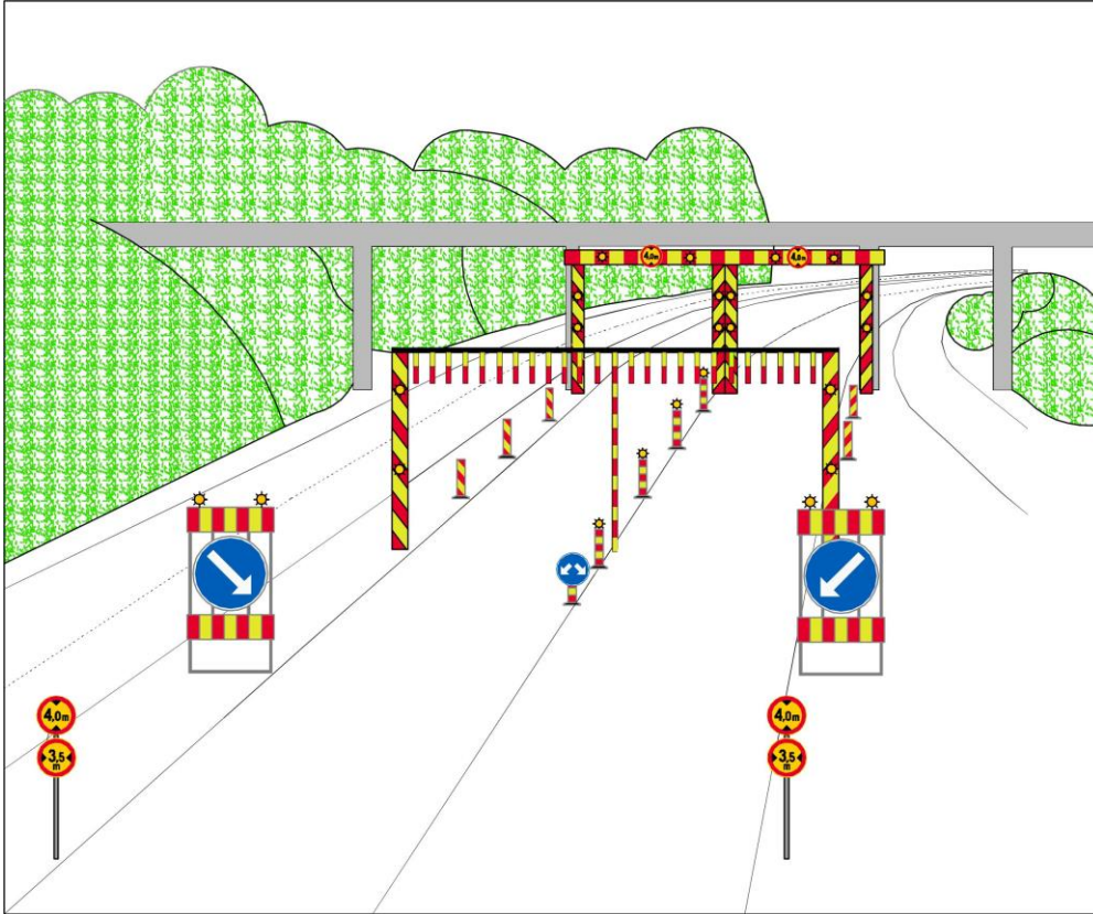
Kuva 17. Esimerkkikuva mittaportista.
