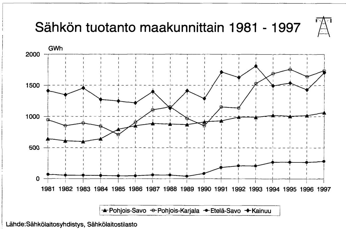
Kuva 110. Sähkön tuotanto maakunnittain 1981 - 1997.
