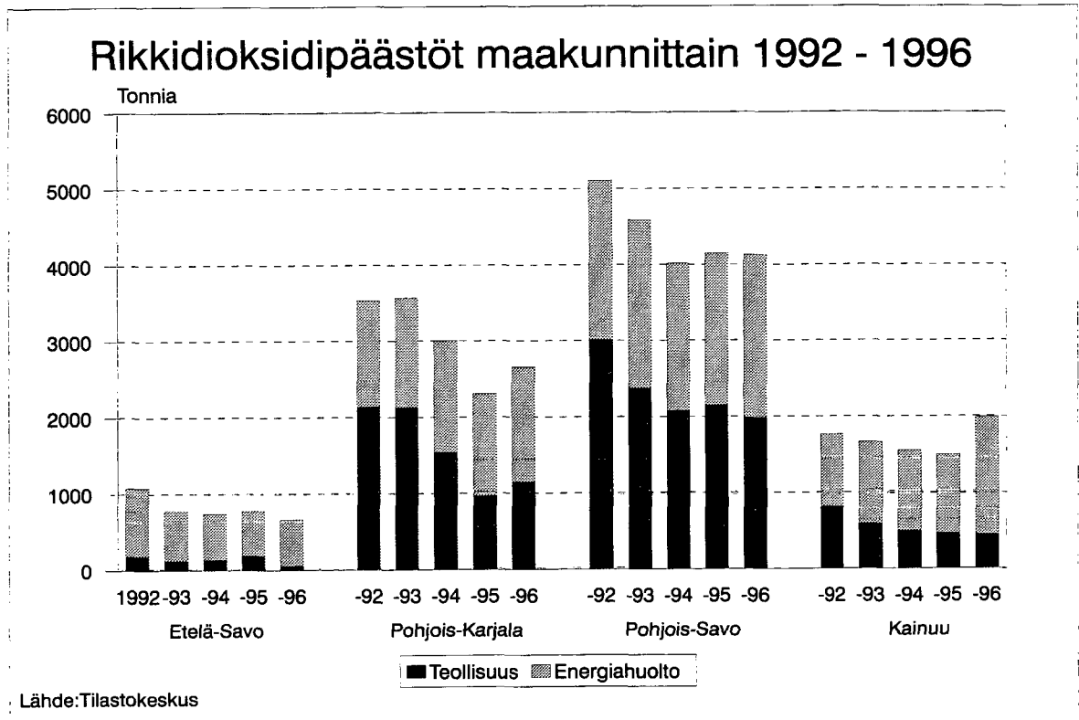
Kuva 118. Rikkidioksidipäästöt maakunnittain 1992 - 1996.
