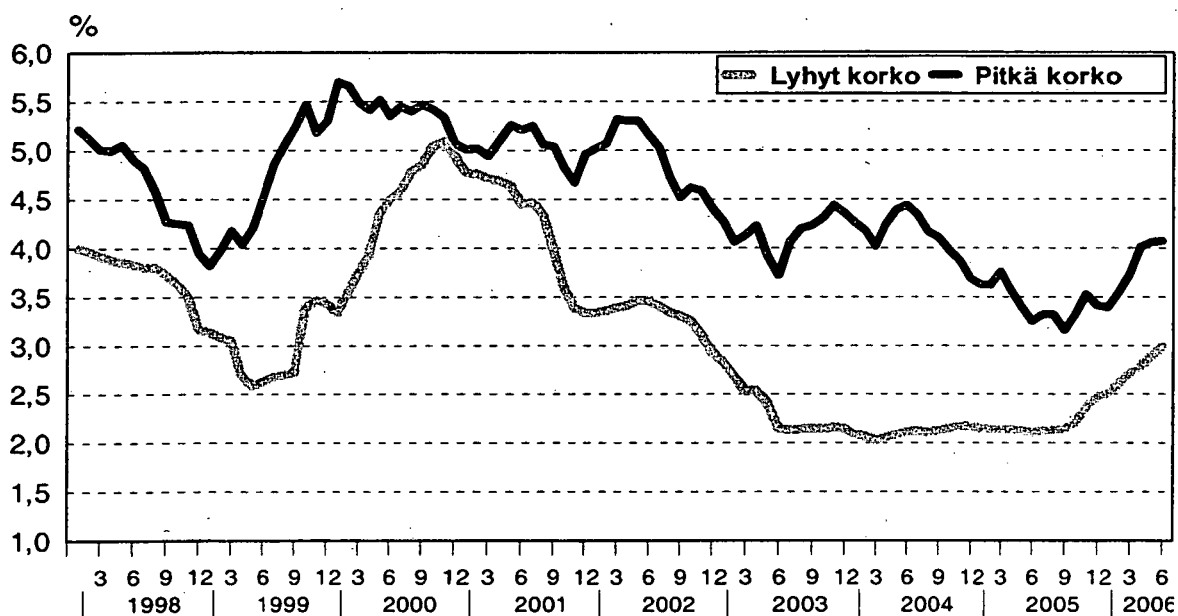
Euroalueen rahamarkkinakorot vuosina 1998 - 2006, %
