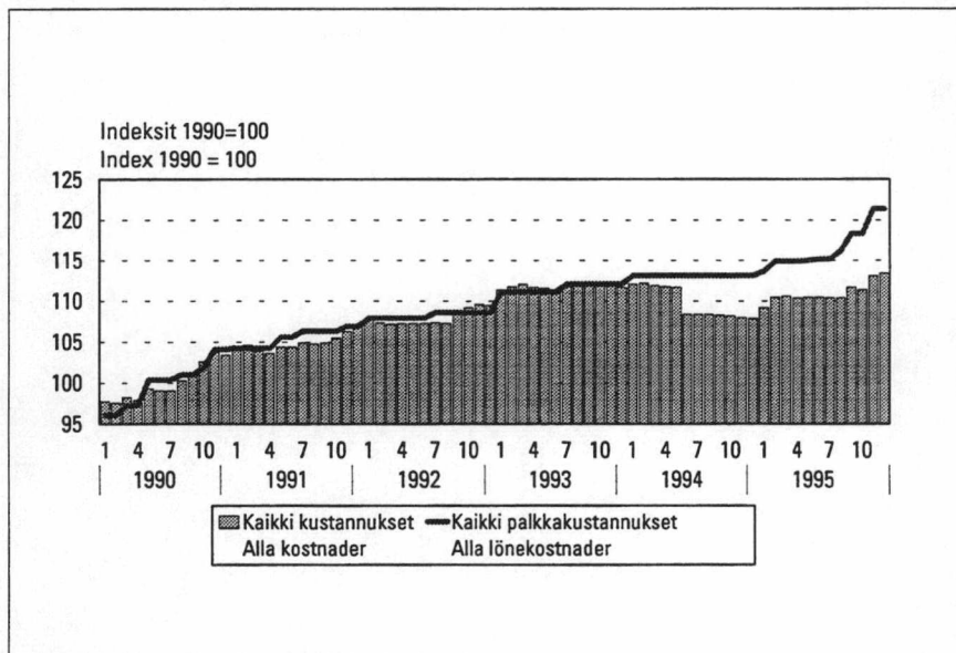
Kuvio 4.2 – Figur 4.2 Linja-autoliikenteen kustannusindeksi (tammi-kuu 1990 – joulukuu 1995) Kostnadsindex för busstrafiken (januari 1990 – december 1995)
