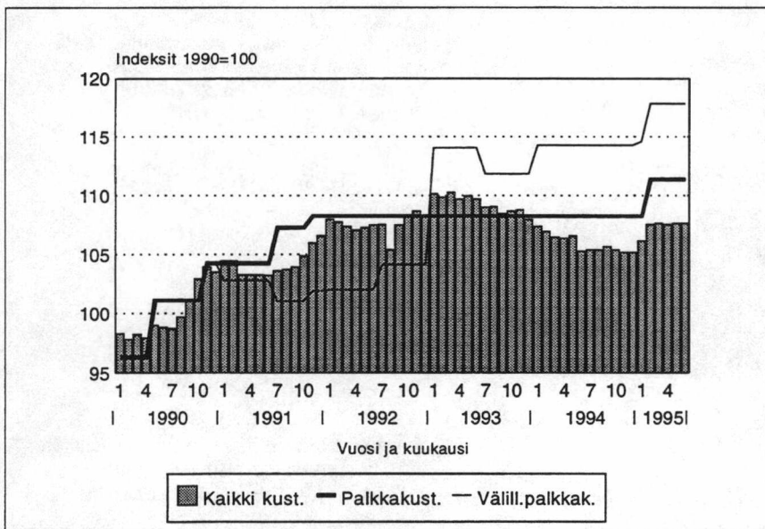
Kuvio 4.1 – Figur 4.1 Kuorma-autoliikenteen kustannusindeksi (tammikuu 1990 – kesäkuu 1995) Kostnadsindex för lastbilstrafiken (januari 1990 – juni 1995)
