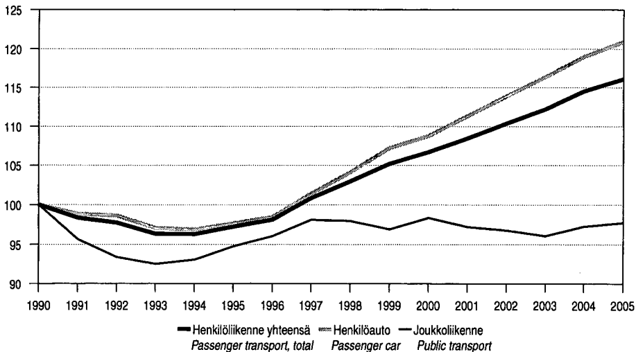
Kuvio 3 – Figure 3 Kotimaan liikenteen henkilökilometriä kehitys (1990=100), 1990–2005 Development of passenger kilometres in domestic transport (1990=100), 1990–2005
