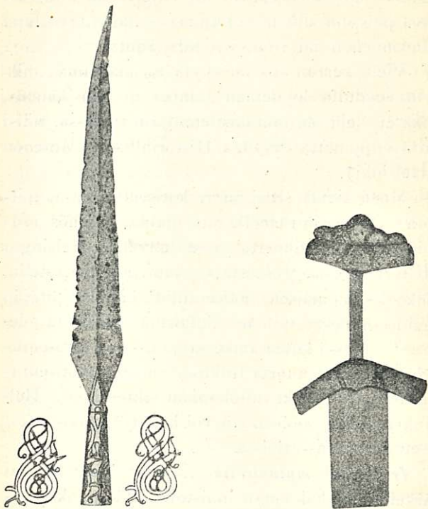
Kuva 6. Muinaisesineitä.
