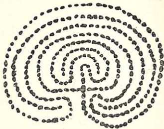
Kuva 4. Jatulintarha.
