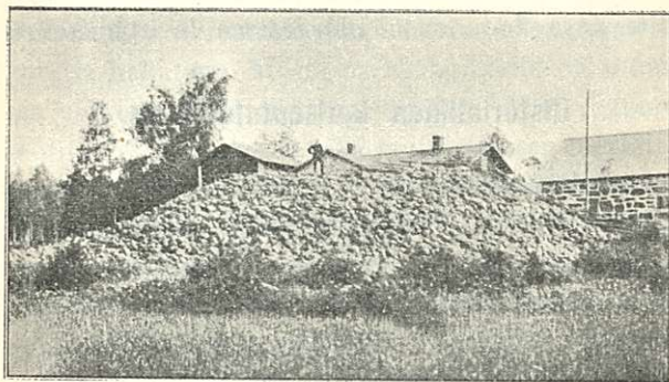
Kuva 2. Hiidenkiuas (Kiukainen).
