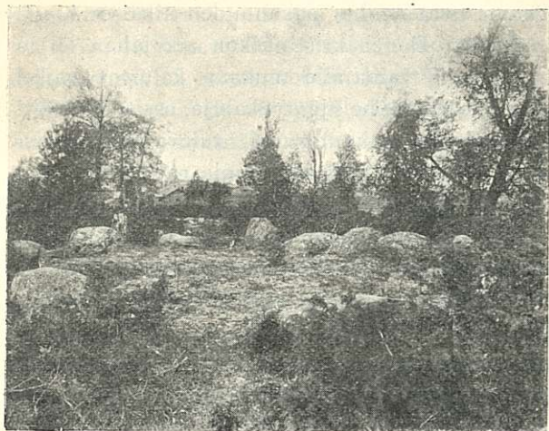
Kuva 5. Tuomarinpiiri.
