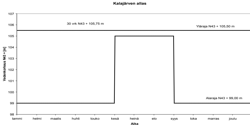
Kuva II. Kalajärven säännöstelyrajat
