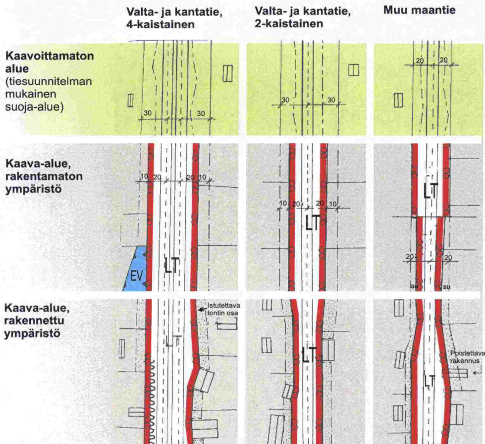
Kuva 11. Periaate liikennealueen rajauksesta sekaliikenneväylillä.
