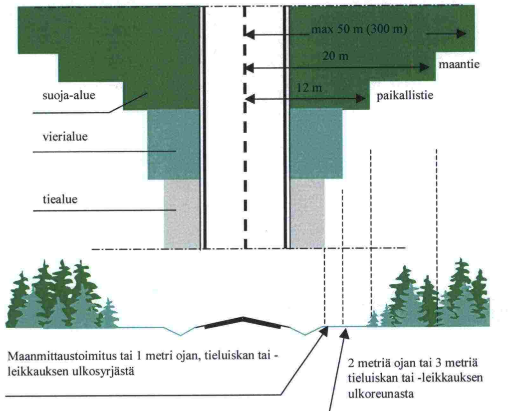
Kuva 10. Tie-, vieri- ja suoja-alueen määrittely.
