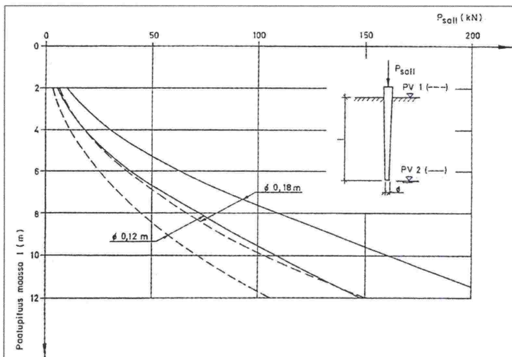
Kuva 28: Puisen kitkapaalun sallittu kokonaiskuorma P_{soll} (kN) löyhässä kitkamaassa, kun kokonaisvarmuuskerroin F = 1,5 . Ehjän viivan (—) arvot pätevät, kun pohjavesi on paalun kärjen tason alapuolella ja katkoviivan (- - -) arvot, kun pohjaveden pinta on paalun kärjen yläpuolella. Siltatelineissä kitkapaalujen varmuuskertoimen tulee kuitenkin olla \geq 2,5 .
