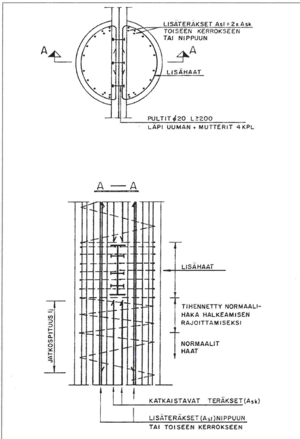
Kuva 38: Pilarin lisäteräket konsolituen yhteydessä
