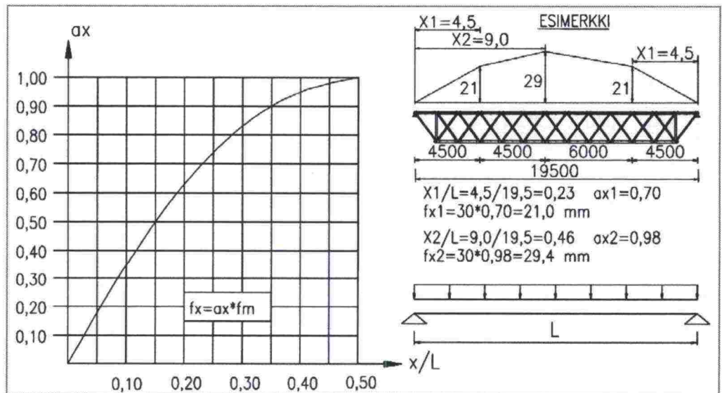
Kuva 34: 1-aukkoisen, tasaisesti kuormitetun kannattimen taipuman f_x määrittäminen välipisteissä, kun tiedetään kannattimen taipuma keskellä f_m = 30 \text{ mm} .
