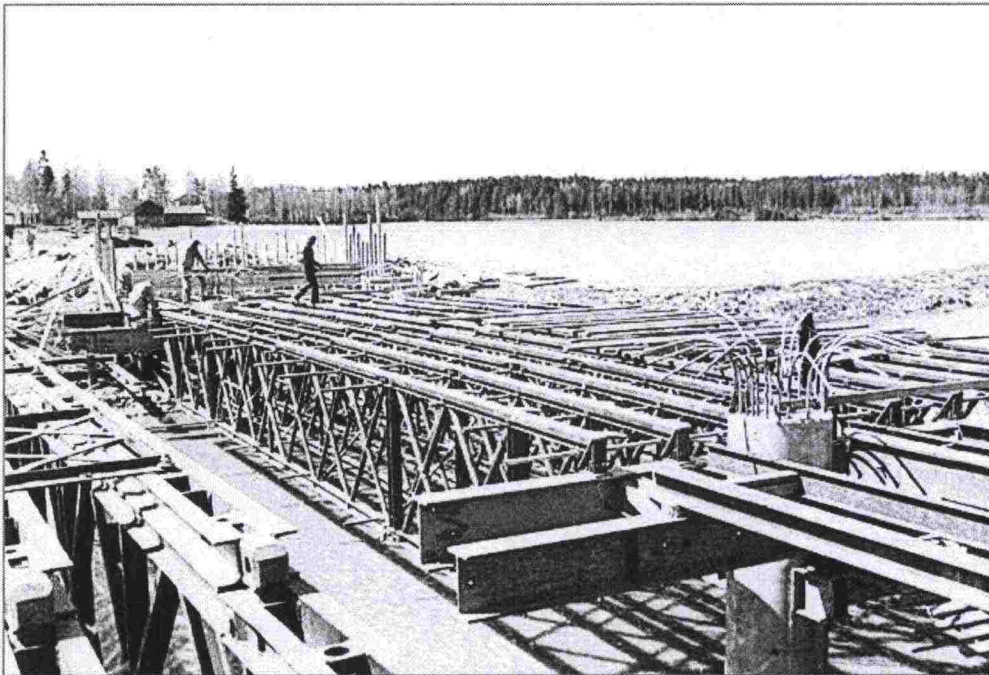
Kuva 41: Kannattimien tuenta pilariin, Mattilan silta
