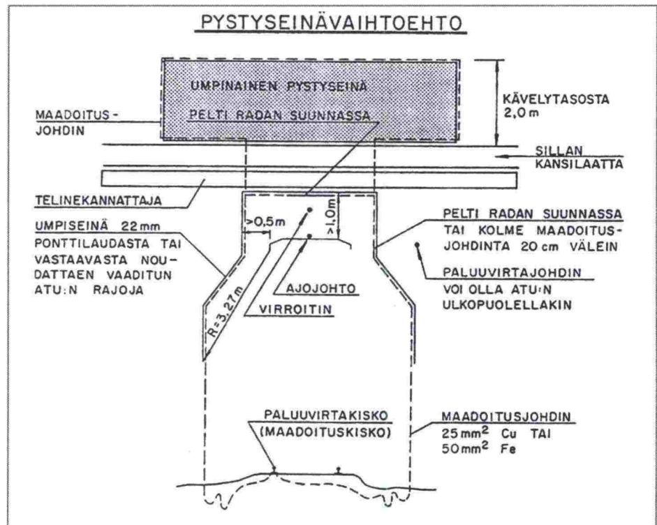
Kuva 50: Ylikulkusillan suojarakenne telineisiin. Pystyseinät sillan reunoilla
