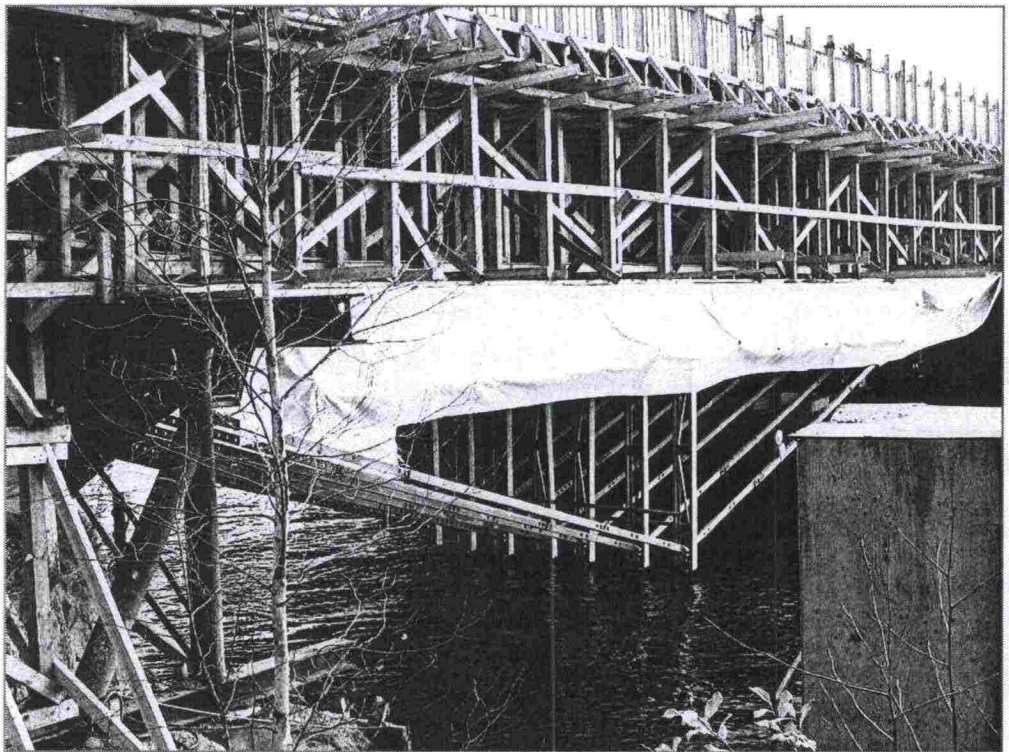
Kuva 14: Peiner V800 kannattimet ja puuteline Vammaskosken sillan korjauksessa
