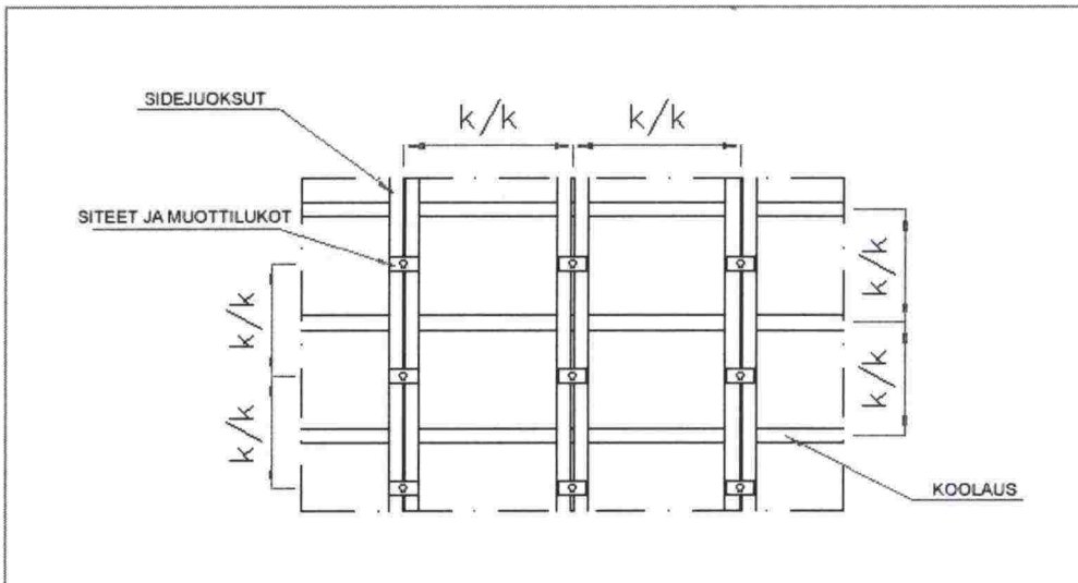
Kuva 54: Periaatekuva seinämuotista
