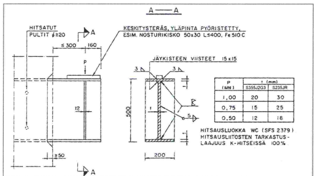
Kuva 37: Levypalkkikonsolin mittoja kuormille P = 0,50 \dots 1,00 MN
