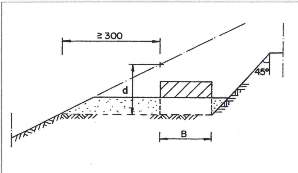
Kuva 25: Perustamissyvyyden määrittäminen luiskassa
