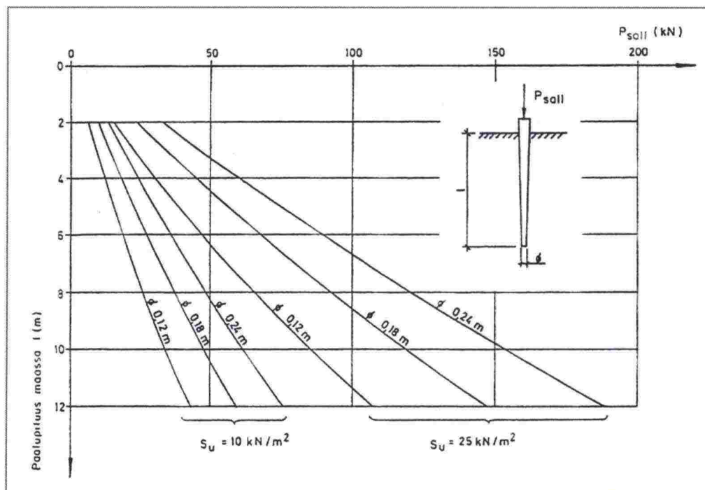
Kuva 29: Puisen koheesiopaalun sallittu kokonaiskuorma P_{soll} (kN) koheesiomaassa S_u \geq 10 \text{ kN/m}^2 , kun kokonaisvarmuuskerroin F = 1,5 . Siltatelineissä tulee varmuuskertoimen olla \geq 2,0 .
