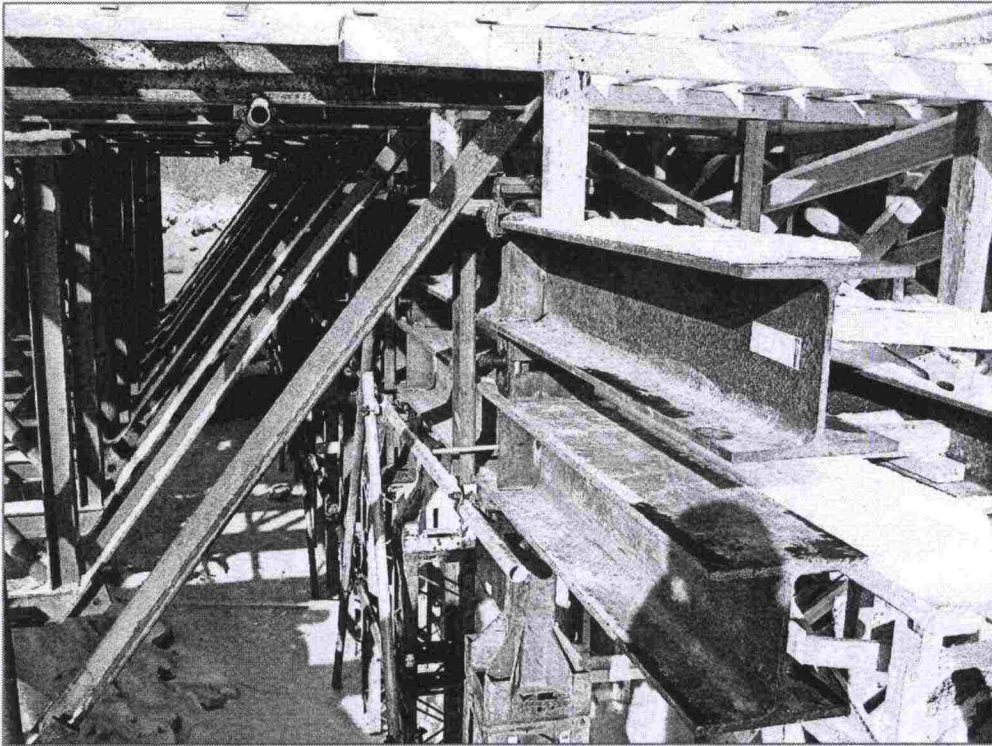
Kuva 11: Hunnebeck H33 kannattimien tuenta
