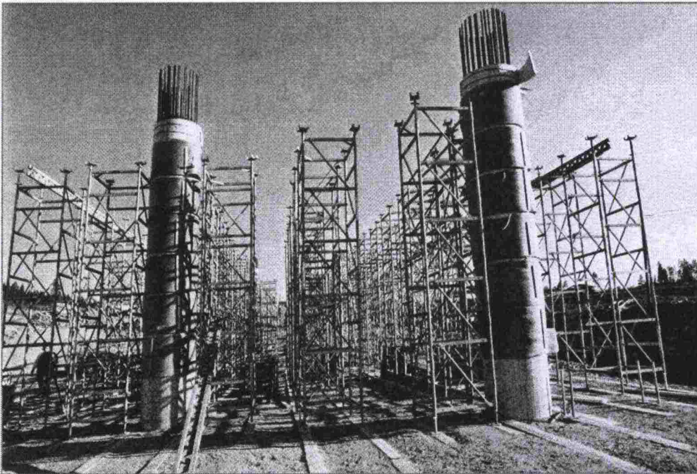
Kuva 12: Kalustotelineitä ja pilarimuotteja
