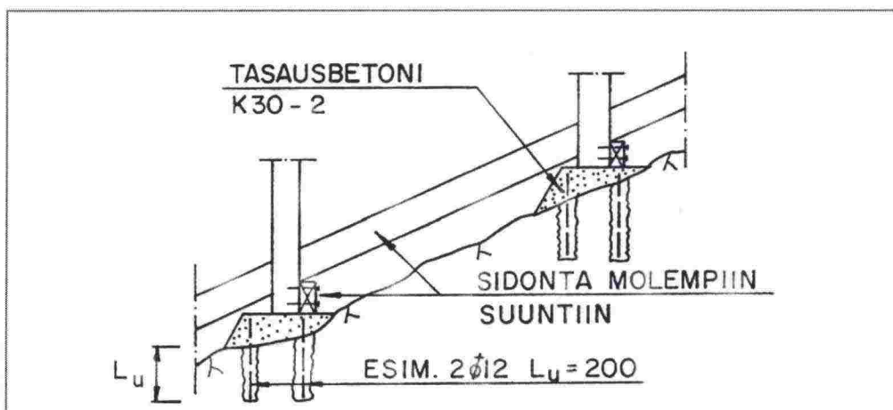
Kuva 26: Perustaminen vinolle kalliopinnalle
