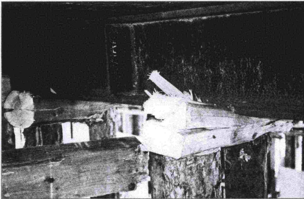
Kuva 5: Leimapaine ylittyy teräspalkin alla
