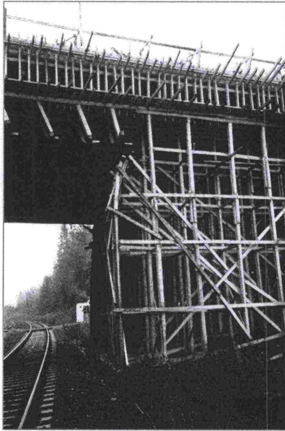
Kuva 3: Riittämätön vinotuenta ja puutteelliset tolppien jatkokset
