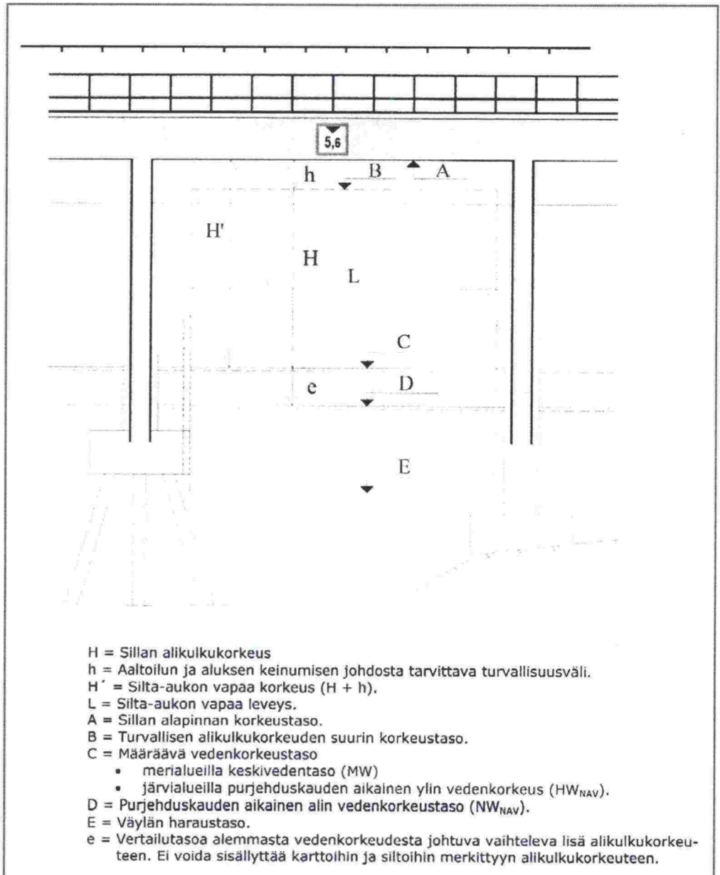
Kuva 52: Vesistösiltojen aukkomittojen määrittely ja käsitteet
