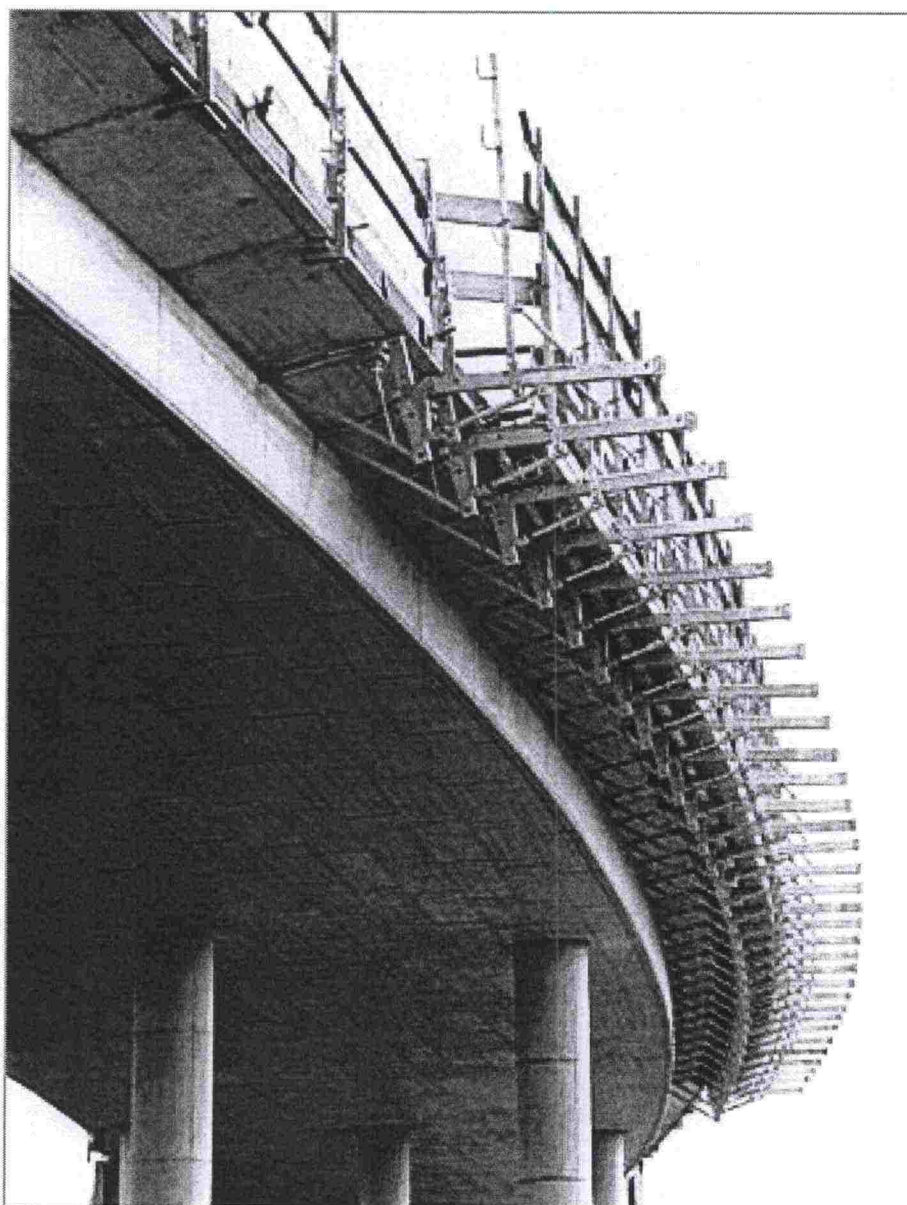
Kuva 46: Reunapalkin korjaus- ja jälkivaluteline
