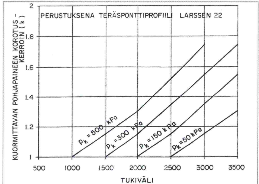
Kuva 21: Kuormittavan pohjapaineen p_{kmax} korotuskertoimet tuen kohdalla tukivälin ja keskimääräisen kuormittavan pohjapaineen funktiona. Perustuksena teräsponsonttiprofiili Larssen 22.
