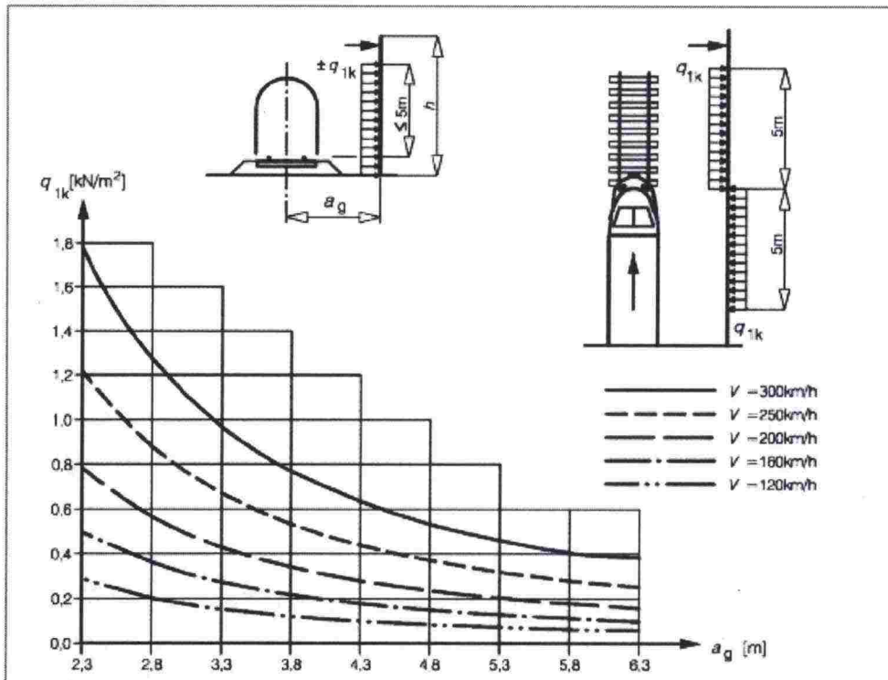
Kuva 17: Raiteen suuntaisten yksinkertaisten pystypintojen kuormien q_{1k} ominaisarvot
