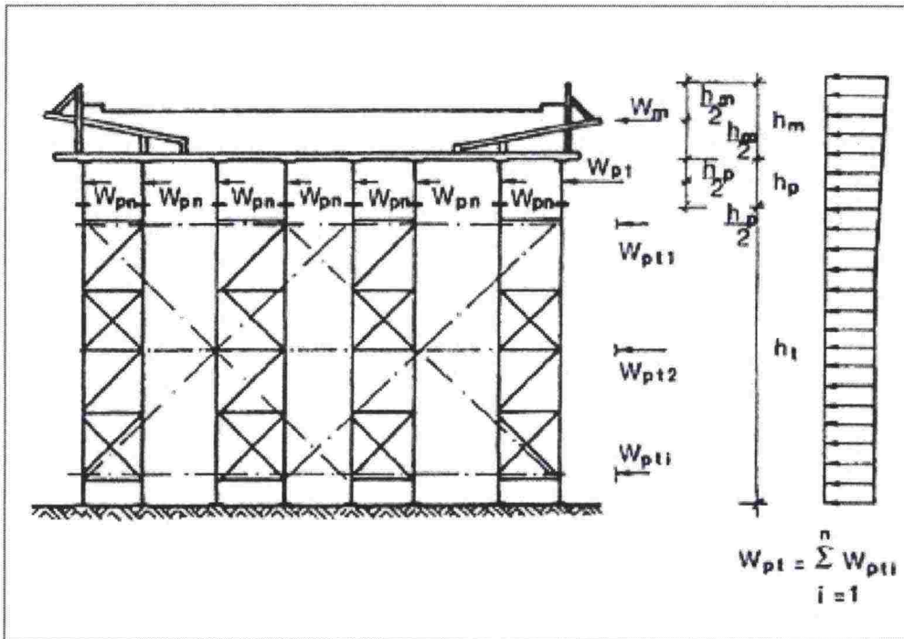
Kuva 16: Tuulikuorma telinekannattimille ja muottiin
