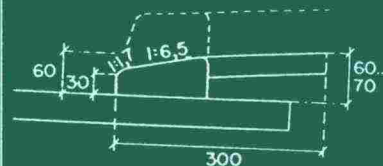
Tb 4 (4a) SUOJATEILLE, JOITA EI OLE TARKOITETTU PYÖRÄILIJÖILLE
