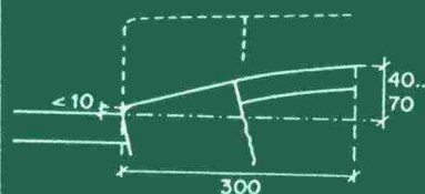
TL 5 [+40] SUOJATEILLE, JOTKA ON TAR- KOITETTU MYÖS PYÖRÄILIJÖILLE.
