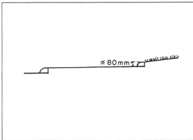
Kuva 5: Jos kevyen liikenteen tien reunassa käytetään reunatukea esim. pintavesien ohjaamiseen tai istutusten suojaamiseen, saa reunatuen korkeus olla enintään 80 mm.
