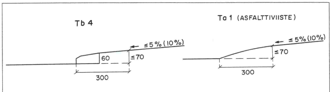
Kuva 3: Kaikkien suojaiteiden kohdalla jalkakäytävän pinta saa kohota ajoradan pinnan jatkeesta 300 mm matkalla enintään 70 mm pyörätuolilla liikkumisen mahdollistamiseksi ja lumen aurauksen helpottamiseksi. Tästä eteenpäin suurin kaltevuus on 10 % ja suositus enintään 5 %.
