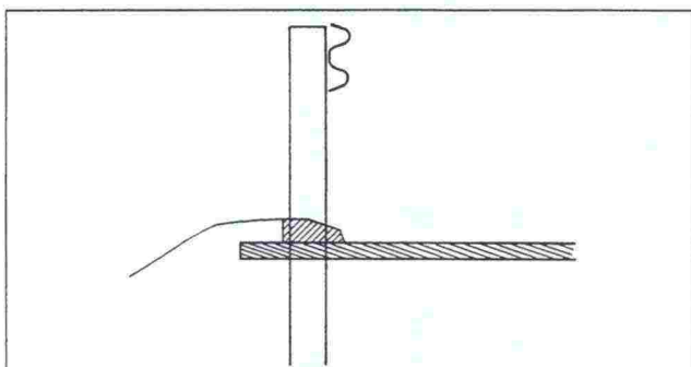
Kuva 6: Jos penkereellä on kaide, reunatuki tulee kaiteen johteen alle. Silloin kaiteen ja reunatuen väliin ei jää vaikeasti jäädä ja roskista puhtaana pidettävää aluetta. Reunatueksi sopii tällöin ma- tala, esimerkiksi asfaltista tehty koroke.
