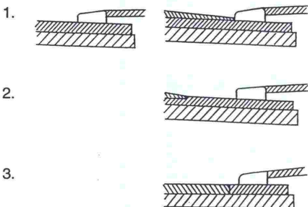
Kuva 7: Ajouradan uudelleenpäällystämisen vaikutus reunatukiin suojatien tai tonttiliittymän kohdalla. Suositeltavin tapa: Aluksi A, myöhemmin D 3.
