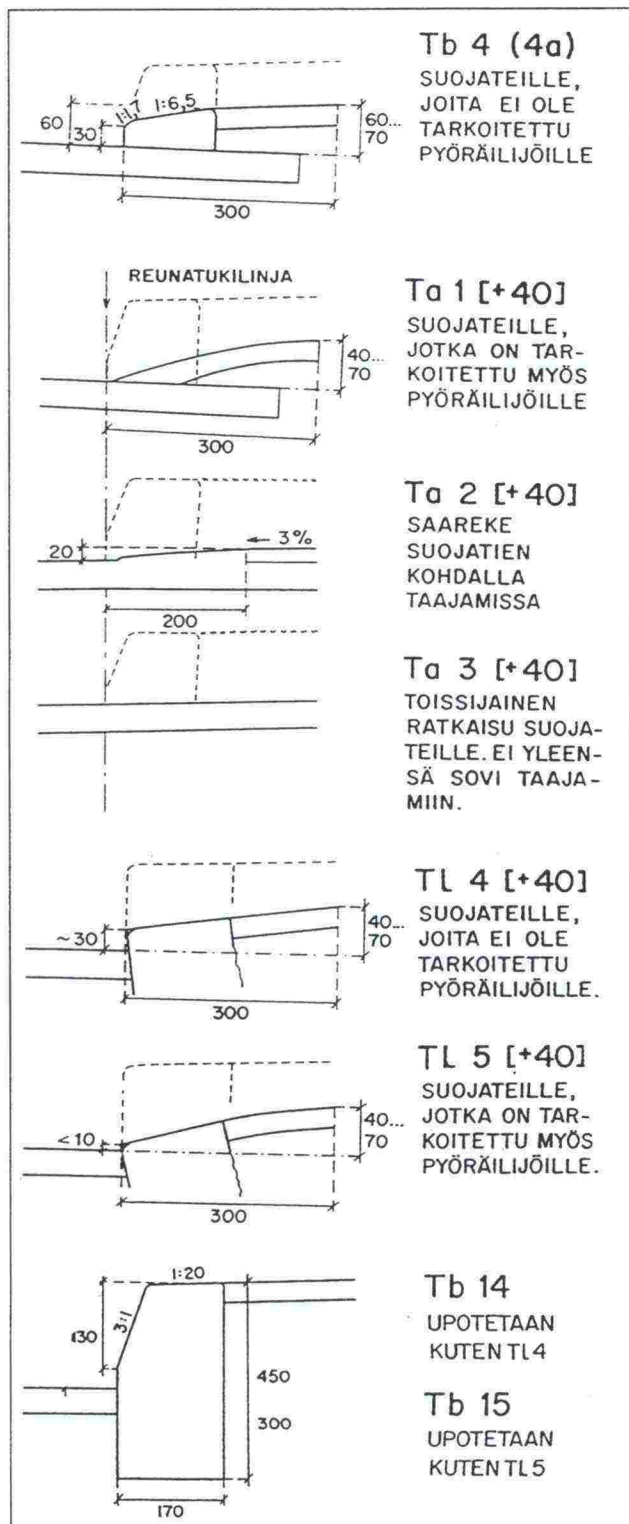
Kuva 4: Suojateillä käytettävät reunatuet ja asfalttiviisteet. Hakasuluissa on mahdollinen korotus vaiheittain rakennettavan päällysteen varalta.
