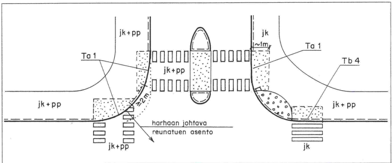
Kuva 2: Reunatuki madalletaan tai korvataan viisteellä 2,5 - 4 m matkalla. Eri suuntien suojaiteiden väliin pitäisi kuitenkin jättää vähintään 2 m täyskorkeaa reunatukea estämään autoja oikaisemasta. Näkövammaisten kulkemisen helpottamiseksi reunatuet tulisi asettaa kohtisuoraan suojatiehen nähden kuten kuvan oikeassa reunassa. Lisäksi suositellaan kohokuvioitua pinnoitetta rasteroidulle alalle alueen tai reitin kaikkien reunatukien kohdalle. Kuvan vasemmassa reunassa kohtisuoruuteen pääsemistä voidaan edistää jättämällä ylitettävän tien keskikoroke pois ja pienentämällä liittymän kaarresäteitä.
