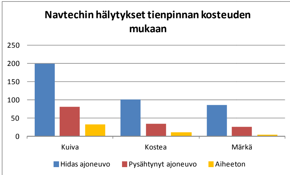
Kuva 42. Navtechin hälytysten määrät tienpinnan kosteuden mukaan.
