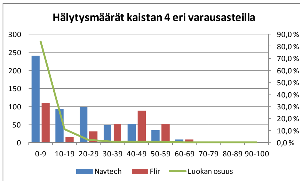
Kuva 55. Hälytysten määrät kaistan 4 eri varausasteluokissa on esitetty pylväillä. Viiva kuvaa varausasteiden jakautumista eri luokkiin pilotin aikana.
