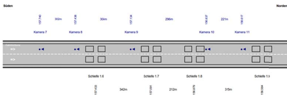
Kuva 10. Elbe-tunnelin testin kameroiden ja silmukoiden sijoitus (LSBG 2012).
