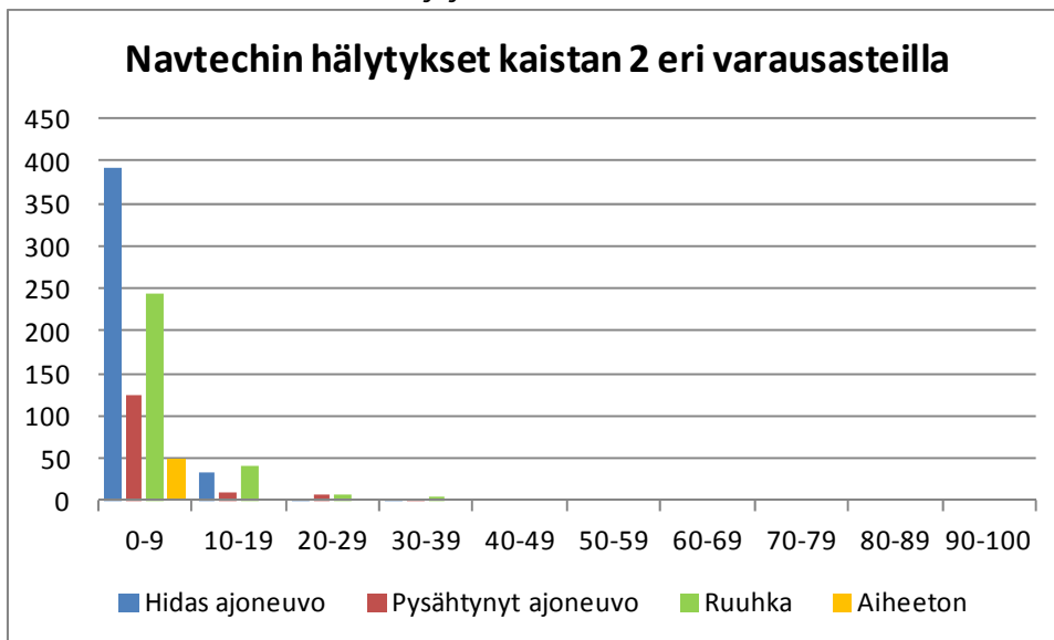
Kuva 51. Navtechin hitaan ja pysähtyneen ajoneuvon hälytysten sekä aiheettomiksi todettujen hälytysten määrät eri varausasteilla kaistalta 2.
