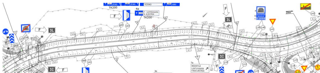
Kuva 11. Ote Mestari-tunnelin liikenteenohjauksen suunnitelmapakartasta (Tiehallinto 25.6.2009).
