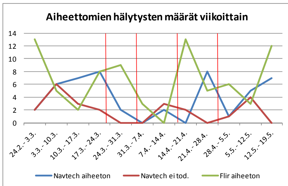
Kuva 58. Navtechin ja Flirin aiheettomien hälytysten ja Navtechin ei todennettavissa olevien hälytysten määrät viikoittain, punaisilla pystyviivoilla merkitty Navtechin järjestelmään tehtyjen merkittävimpien muutosten ajankohdat.
