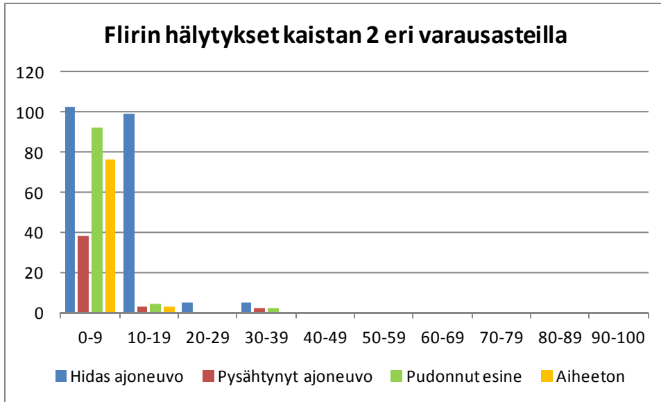
Kuva 50. Flirin tekemien hitaan ja pysähtyneen ajoneuvon ja pudonneen esineen hälytysten määrät sekä aiheettomiksi todettujen hälytysten määrät eri varausasteilla kaistalta 2.
