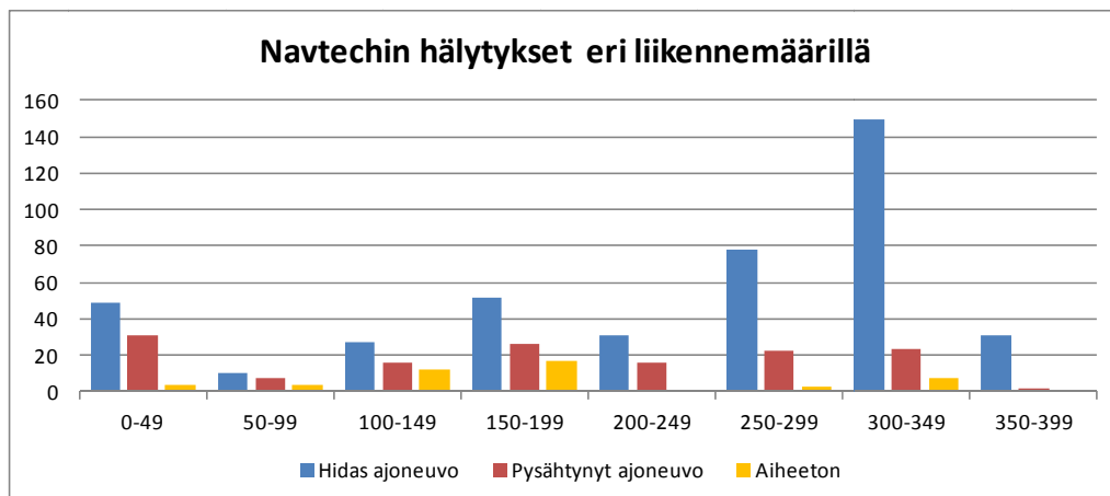
Kuva 45. Navtechin hitaan ja pysähtyneen ajoneuvon hälytysten sekä aiheettomiksi todettujen hälytysten määrät eri liikennemääräluokissa.
