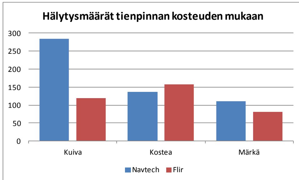
Kuva 40. Hälytysten määrät tienpinnan eri kosteusasteilla.
