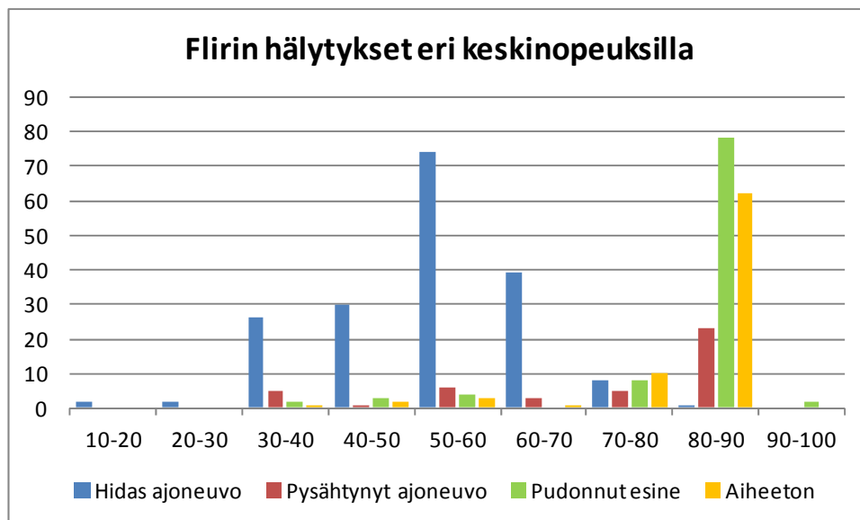
Kuva 47. Flirin tekemien hitaan ja pysähtyneen ajoneuvon ja pudonneen esineen hälytysten määrät sekä aiheettomiksi todettujen hälytysten määrät eri keskinopeusluokissa.
