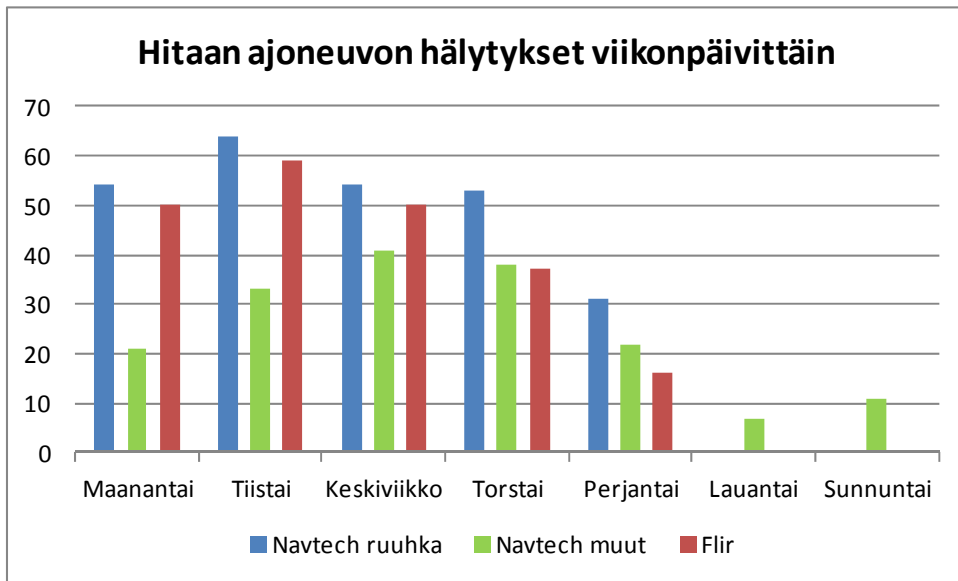
Kuva 21. Hitaan ajoneuvon hälytysten määrät viikonpäivittäin.
