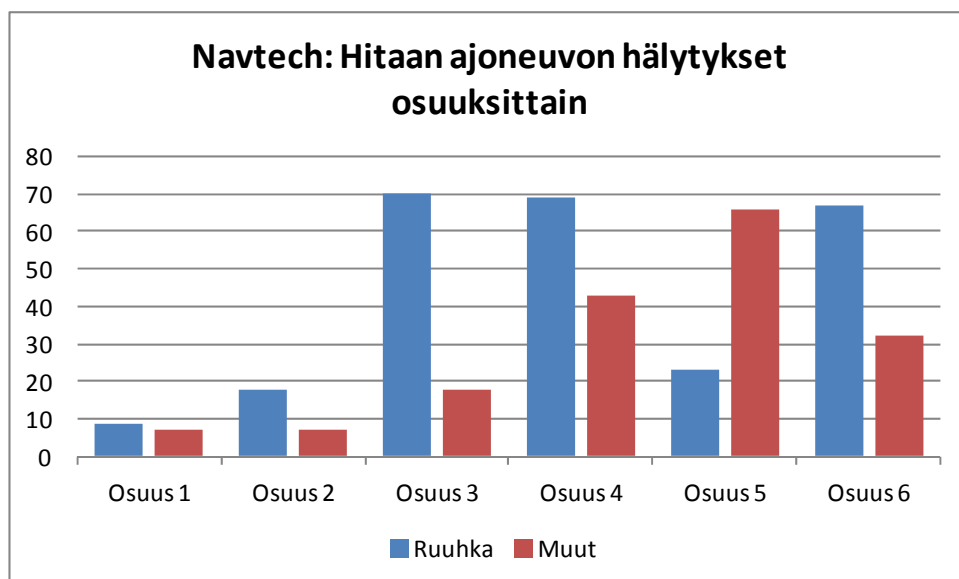
Kuva 20. Navtechin ruuhkasta ja muista syistä aiheutuneet hitaan ajoneuvon hälytykset havainto-osuuksittain (yht. 429 kpl).
