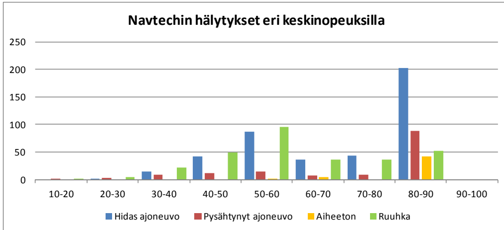
Kuva 48. Navtechin hitaan ja pysähtyneen ajoneuvon hälytysten sekä aiheettomiksi ja ruuhkasta aiheutuneiksi todettujen hälytysten määrät eri keskinopeusluokissa.
