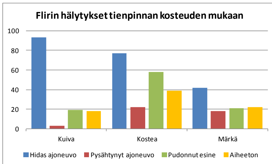
Kuva 41. Flirin hälytysten määrät tienpinnan eri kosteusasteilla.
