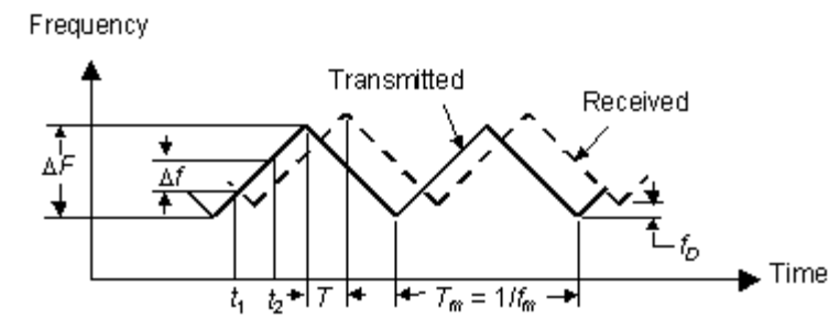
Kuva 4. Taajuusmodulaatiota käyttävän tutkan toimintaperiaate (FHWA 2015)
