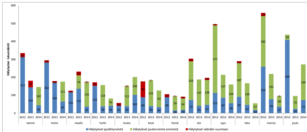
Kuva 6. Mestarintunnelin HHJ-hälytysten määrät kuukausittain 2012–2014. Pysähtyneen ajoneuvon hälytykset ovat kuvaajassa sinisellä (alimmaisena), pudonneen esineen hälytykset vihreällä (keskimmäisenä) ja väärään suuntaan ajavan hälytykset punaisella (ylimpänä). (Uudenmaan ELY-keskus 2015.)
