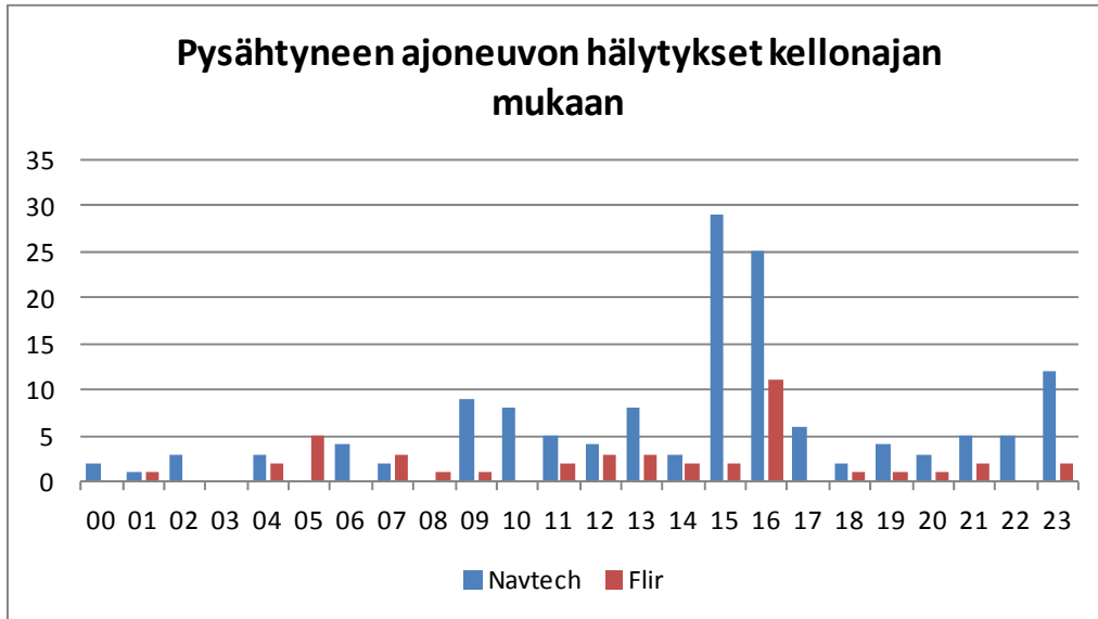
Kuva 28. Pysähtyneen ajoneuvon hälytysten määrät kellonajan mukaan. Vaakakselilla alkavat tunnit.
