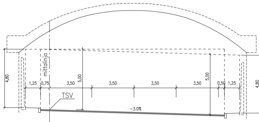
Kuva 13. Mestarintunnelin itäisen ajoradan poikkileikkaus plv. 6565–6770.
