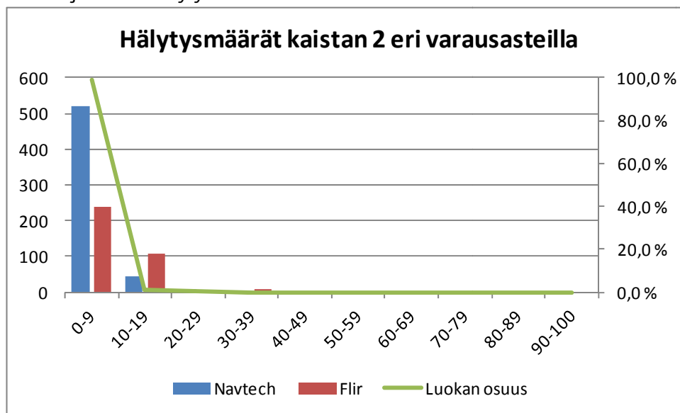
Kuva 49. Hälytysten määrät kaistan 2 eri varausasteiluokissa on esitetty pylväillä. Viiva kuvaa varausasteiden jakautumista eri luokkiin pilotin aikana.
