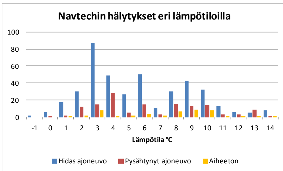
Kuva 36. Navtechin tekemät hitaan ja pysähtyneen ajoneuvon sekä aiheettomiksi todettujen hälytysten määrät eri ilman lämpötiloilla (tiesääasema Mestarintunneli R_1092).
