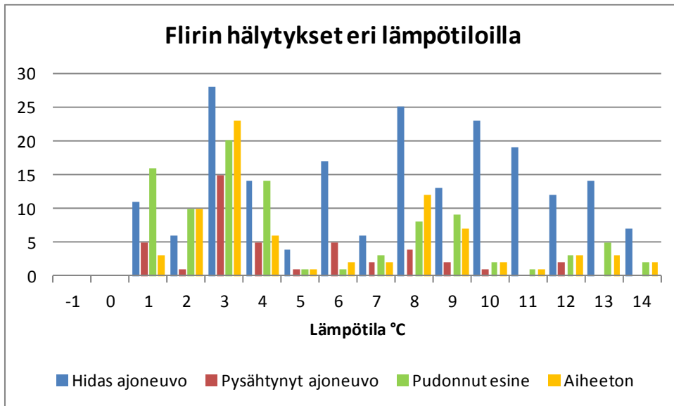
Kuva 35. Flirin tekemät hitaan ja pysähtyneen ajoneuvon ja pudonneen esineen hälytysten sekä aiheettomiksi todettujen hälytysten määrät eri ilman lämpötiloilla (tiesääasema Mestarintunneli R_1092).
