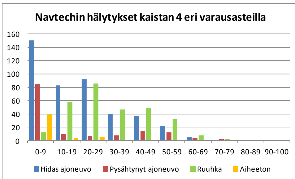
Kuva 57. Navtechin hitaan ja pysähtyneen ajoneuvon hälytysten sekä ruuhkasta aiheutuneiksi ja aiheettomiksi todettujen hälytysten määrät eri varausasteilla kaistalta 4.
