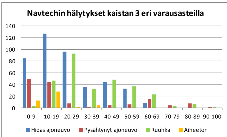
Kuva 54. Navtechin hitaan ja pysähtyneen ajoneuvon hälytysten sekä ruuhkasta aiheutuneiksi ja aiheettomiksi todettujen hälytysten määrät RTJ103 eri varausasteilla kaistalta 3.
