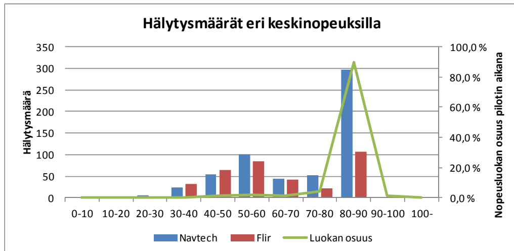
Kuva 46. Hälytysten määrät eri 5 min keskinopeuksilla on esitetty pylväillä. Viiva kuvaa 5 min jaksojen keskinopeuksien jakautumista eri luokkiin pilotin aikana.
