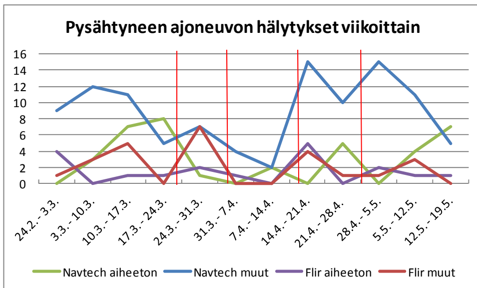
Kuva 31. Pysähtyneen ajoneuvon hälytykset viikoittain. Punaisilla pystyviivoilla merkitty Navtechin järjestelmään tehtyjen merkittävimpien muutosten ajankohdat.
