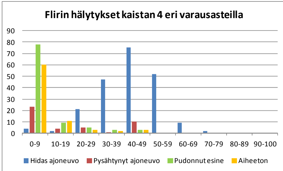
Kuva 56. Flirin hitaan ja pysähtyneen ajoneuvon ja pudonneen esineen hälytysten määrät sekä aiheettomiksi todettujen hälytysten määrät eri varausasteilla kaistalta 4.
