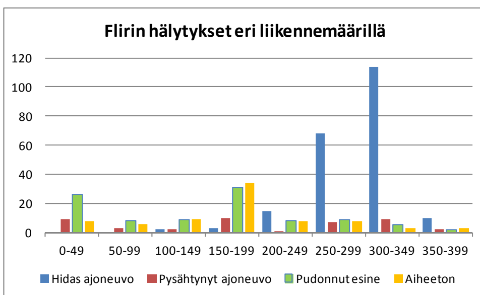
Kuva 44. Flirin tekemien hitaan ja pysähtyneen ajoneuvon ja pudonneen esineen hälytysten määrät sekä aiheettomiksi todettujen hälytysten määrät eri liikennemääräluokissa.
