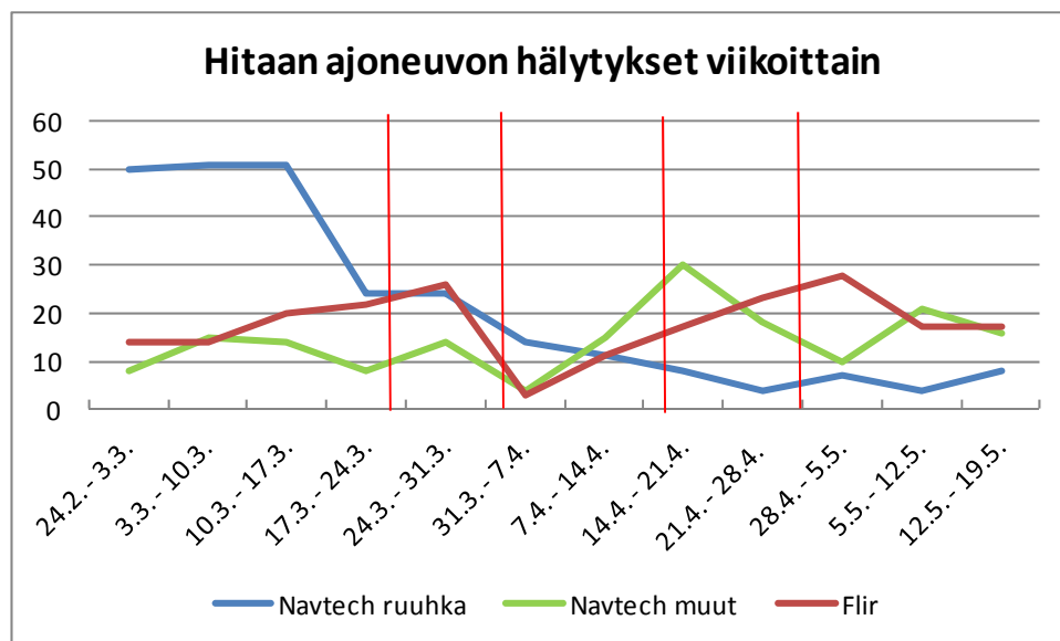
Kuva 23. Hitaan ajoneuvon hälytykset viikoittain, punaisilla pystyviivoilla on merkitty Navtechin järjestelmään tehtyjen merkittävimpään asetusten ajankohdat.
