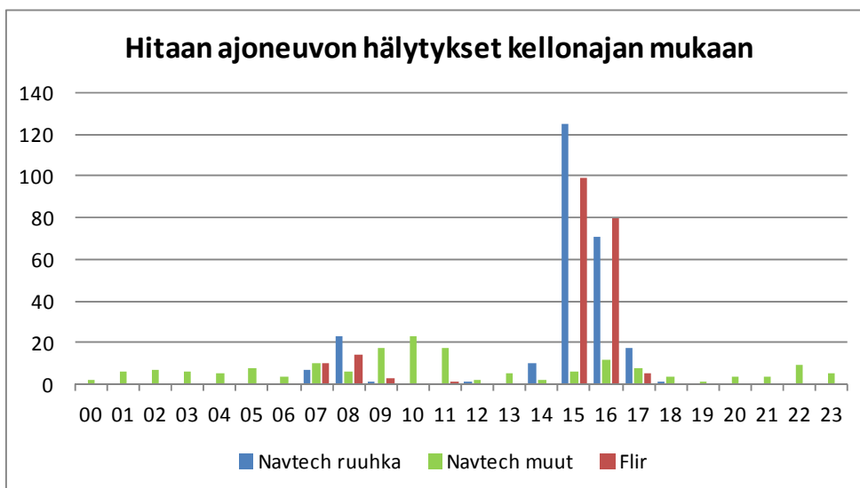
Kuva 22. Hitaan ajoneuvon hälytysten määrät kellonajan mukaan. Vaakselilla alkavat tunnit.
