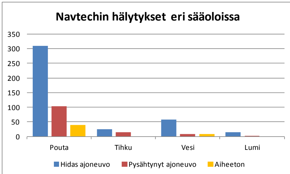
Kuva 39. Navtechin tekemät hitaan ja pysähtyneen ajoneuvon sekä aiheettomiksi todettujen hälytysten määrät eri sääoloissa (tiesäasema Vallikallio R_1096).
