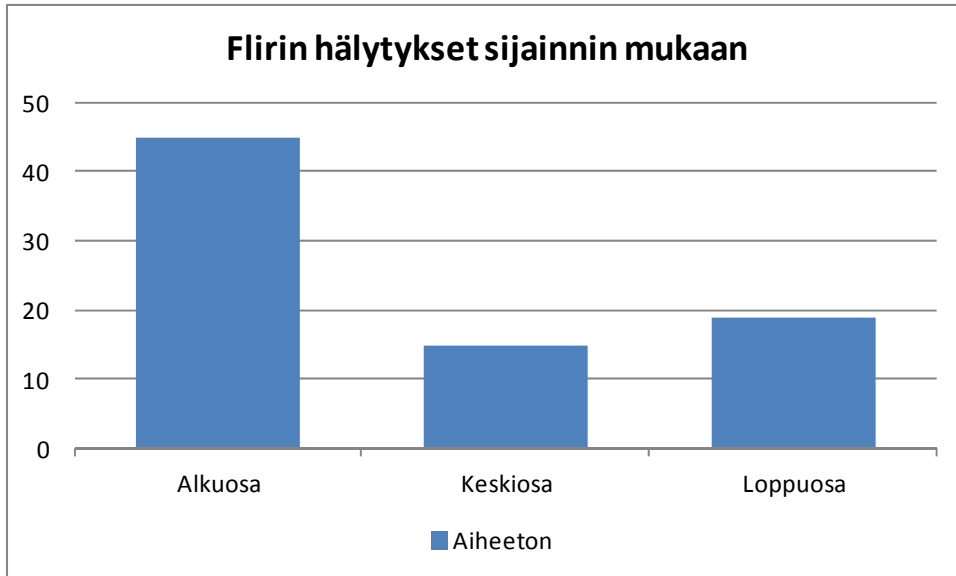
Kuva 59. Flirin aiheettomien hälytysten määrät tunnelin eri osissa.
