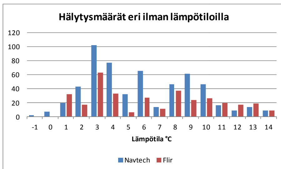
Kuva 34. Hälytysmäärät eri ilman lämpötiloilla (tiesääasema Mestarintunneli R_1092).
