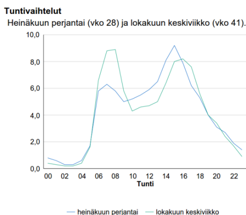
Kuva 12. Konalan LAM-pisteen (nro 126) tuntivaihtelut 2014 (Liikennevirasto 2015b).
