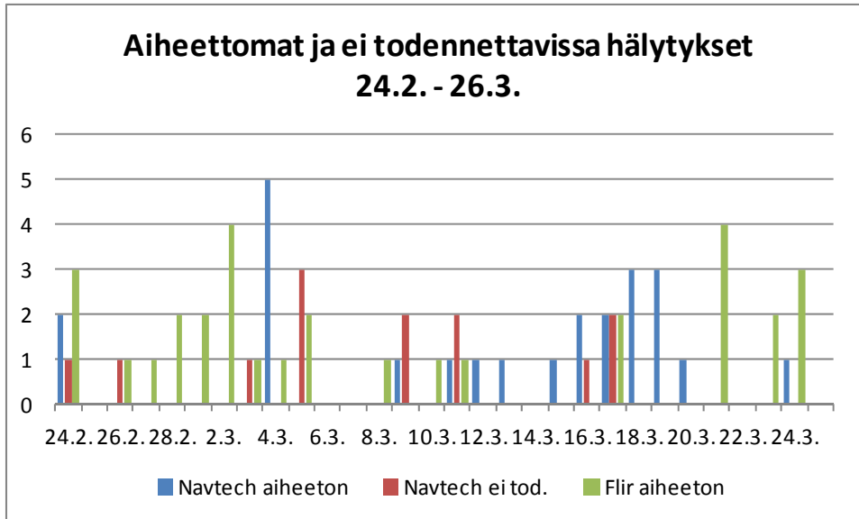
Kuva 62. Pilotin ensimmäisen 30 päivän aiheettomat ja ei todennettavissa olevien hälytysten määrät.
