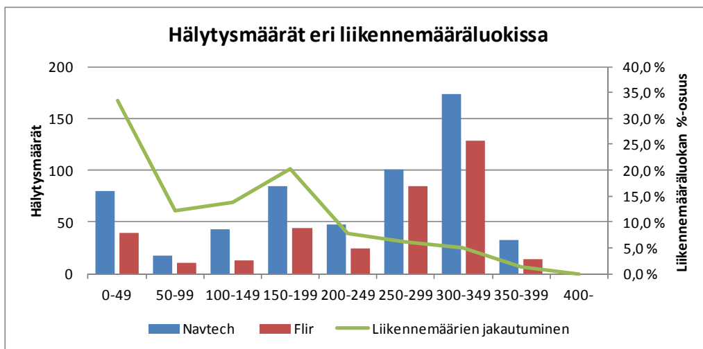
Kuva 43. Hälytysten määrät eri 5 min liikennemääräluokissa on esitetty pylväillä. Viiva kuvaa 5 min jaksojen liikennemäärien jakautumista eri luokkiin pitkin aikaa.
