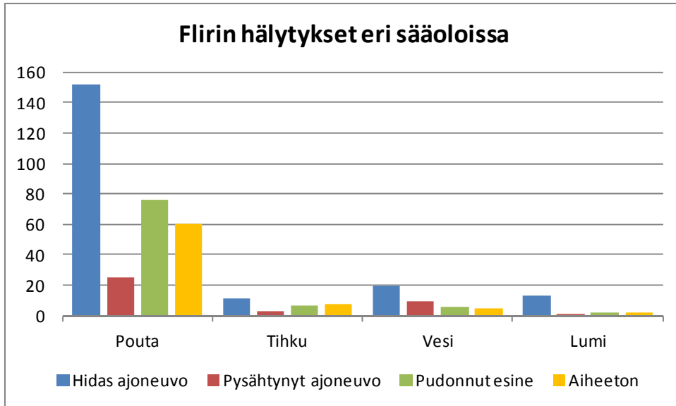
Kuva 38. Flirin tekemien hitaan ja pysähtyneen ajoneuvon ja pudonneen esineen hälytysten sekä aiheettomiksi todettujen hälytysten määrät eri sääoloissa (tiesäasema Vallikallio R_1096).
