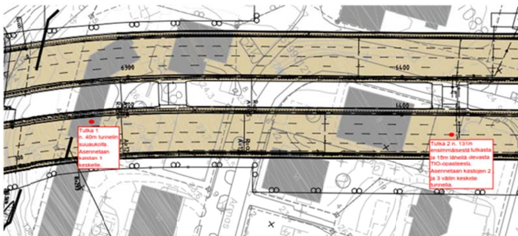
Kuva 14. Tutkien 1 ja 2 sijoituspaikat (YSP 2015).
