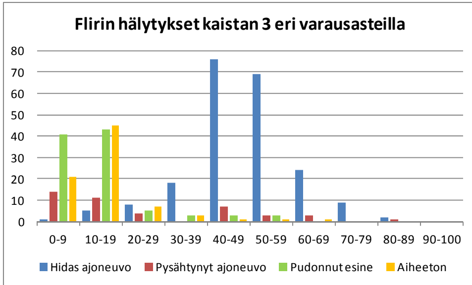
Kuva 53. Flirin hitaan ja pysähtyneen ajoneuvon ja pudonneen esineen hälytysten määrät sekä aiheettomiksi todettujen hälytysten määrät RTJ103 eri varausasteilla kaistalta 3.
