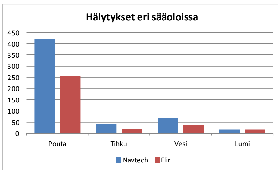
Kuva 37. Hälytysten määrät eri sääoloissa (tiesääasema Vallikallio R_1096).
