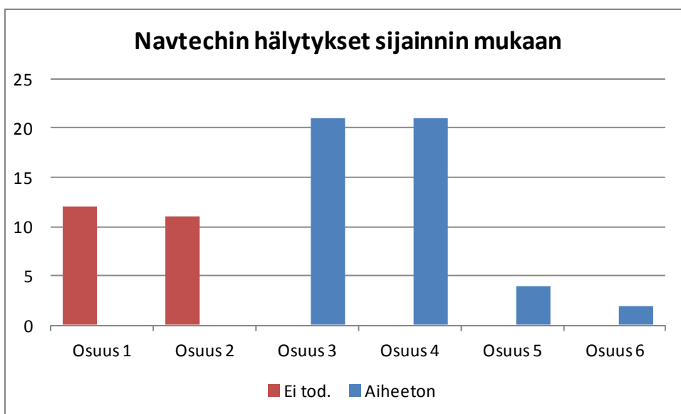
Kuva 60. Navtechin aiheettomien ja ei todennettavissa olevien hälytysten määrät sijainnin mukaan.
