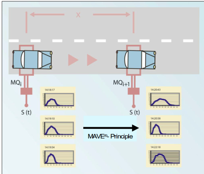
Kuva 5. Ajoneuvojen tunnistus MAVE-tunin järjestelmässä (Böhnke 2011).
