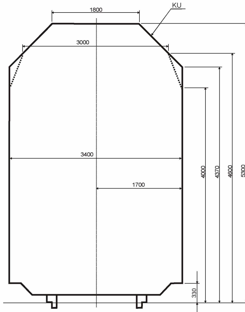
Kuva 9. Kuormaulottuma.
