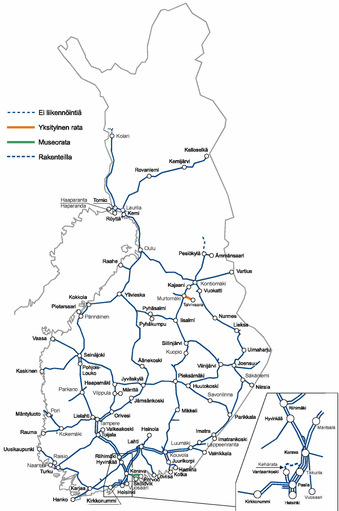
Kuva 1. Rataverkko
