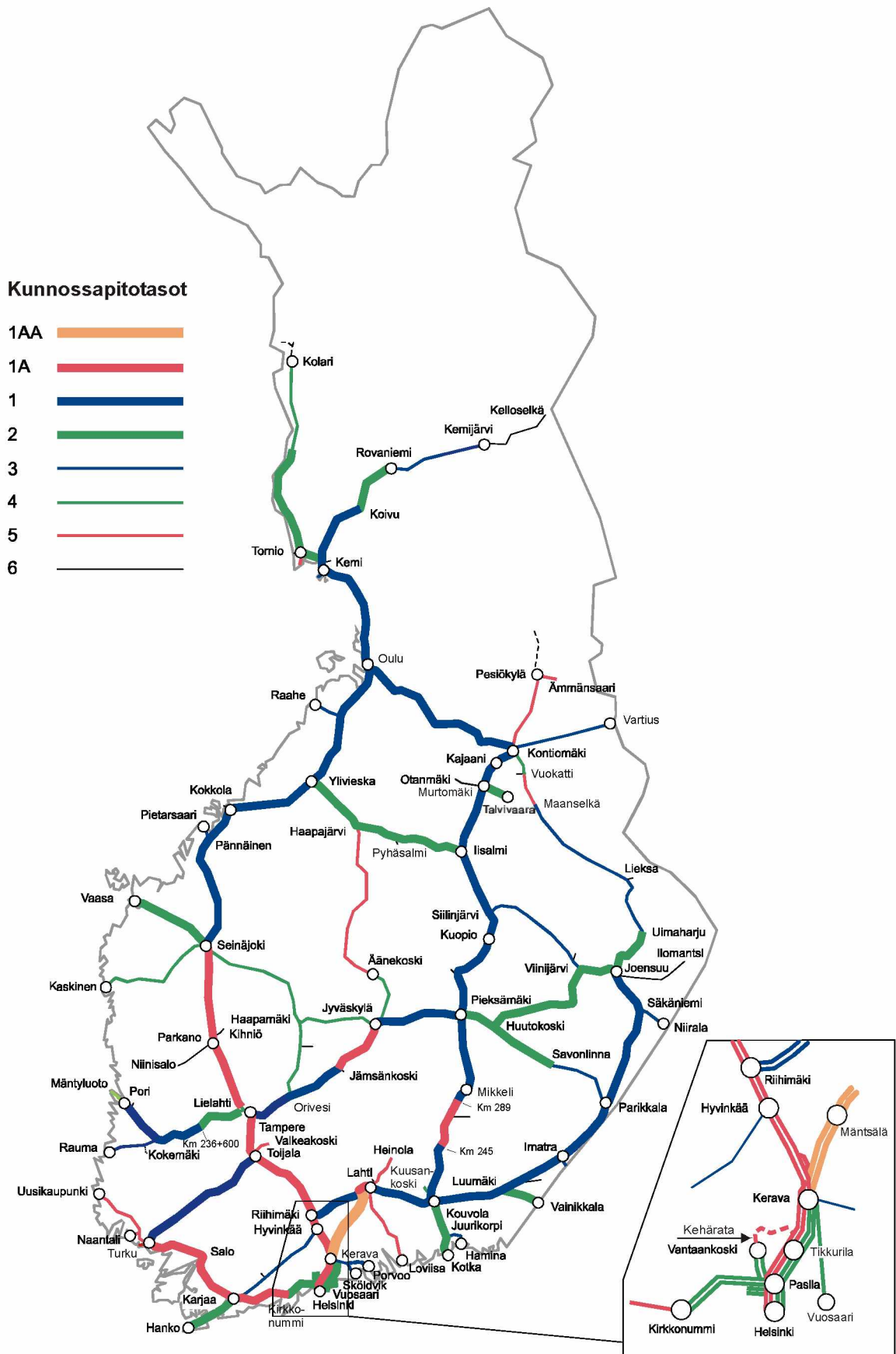
Kuva 2. Pääratojen kunnossapitotasot
