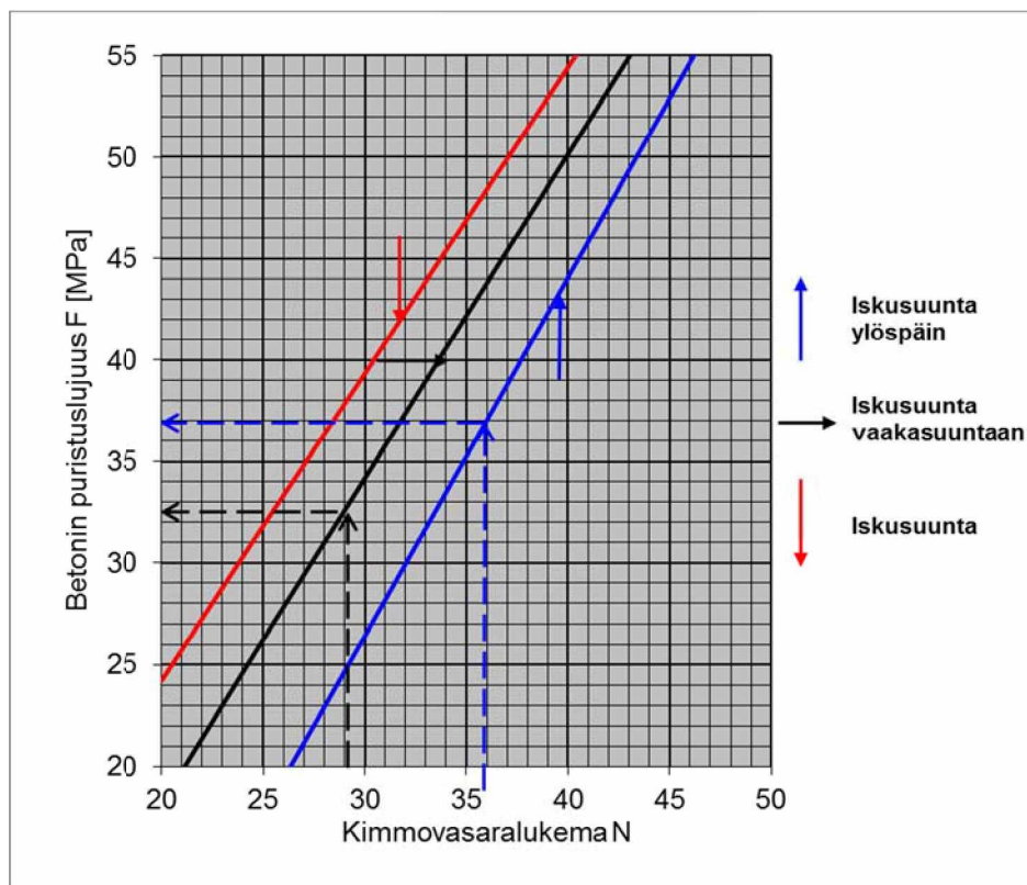
Kuva 1. Testauskohdan puristuslujuuden ja kimmovasaralukeman välinen yleinen riippuvuus.
