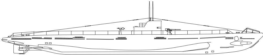
ETEHNEN, Suomi 1930. Pituus 63 m, uppouma 493/716 t, miehistö 30, aseistus 4 torpedoputkea, 20 miinaa, 76 mm:n tykki, 20 mm:n konekytkki. Romutettu 1953.
