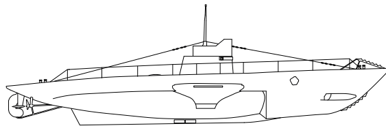
AUKKO, Suomi 1930. Pituus: 33 m, uppouma 99/150 t, miehistö 15, aseistus: 2 torpedoputkea, 9 miinaa. Romutettu 1953.
