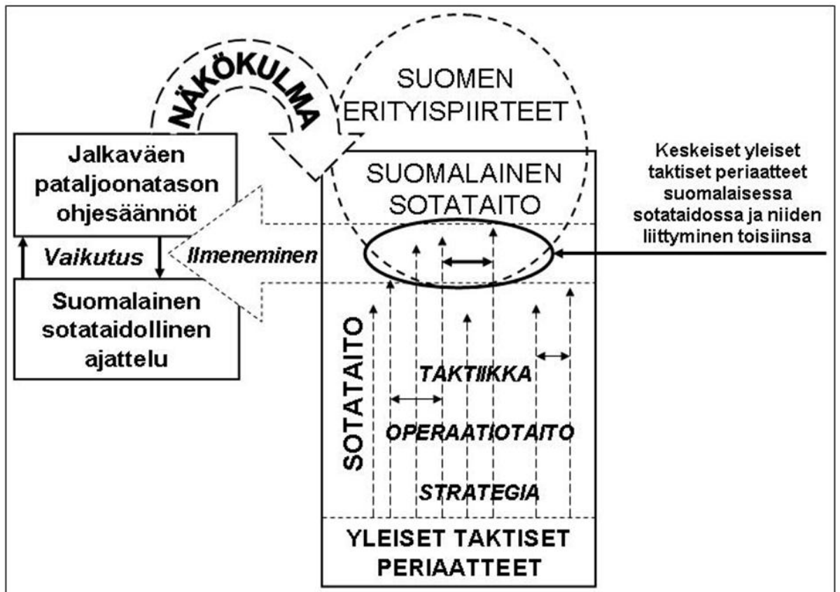
Kuva 1. Tutkimuksen viitekehys.
