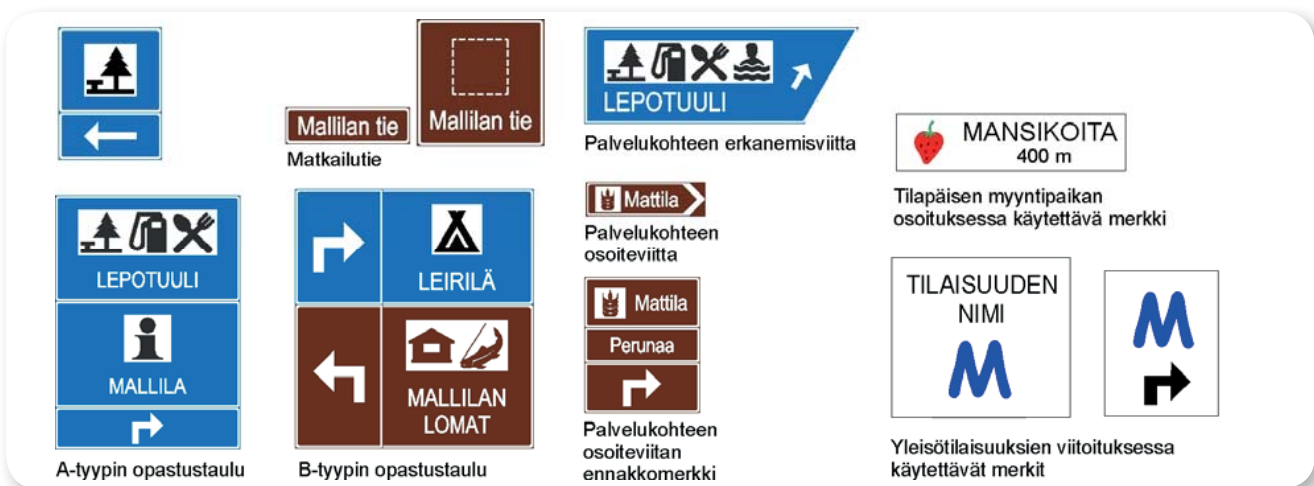
Kuva 1-2. Palvelukohteen viitoituksessa käytettävät liikennemerkit.
