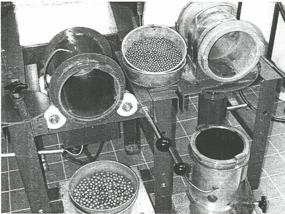
Kuva 2. Kuulamylylaite (vas.), normaali Micro-Deval-rumpu (ylh.oik.), raideseppelin testaamisessa käytettävä Micro-Deval-rumpu (alh. oik.) ja kokeissa käytettävät kuulat.
