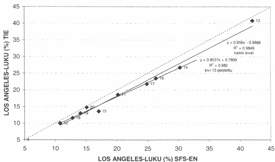
Kuva 4. SFS-EN- ja TIE-menetelmillä määritettyjen Los Angeles -lukujen välinen riippuvuus.
