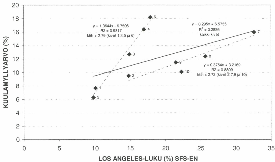
Kuva 8. Los Angeles -luvun (SFS-EN) ja kuulamylyarvon välinen riippuvuus.
