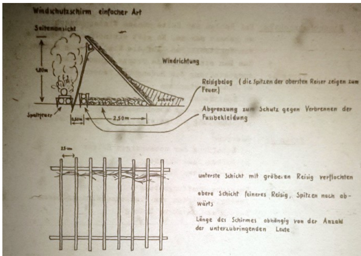
Kuva 2: Saksalaisen 36. Vuoristoarmeijakunnan esikunnan ohje partion tilapäismajoittumiseen. Ohje ovat hyvin samanlainen kuin vuonna 1928 julkaistussa Talvisotakäsikirjassa ja Päämajan muistiossa PM:n kaukopartioinnista talvella . 70
