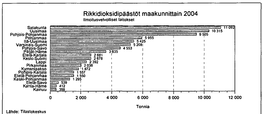
Kuva 18.7. Rikkidioksidipäästöt maakunnittain 2004.
