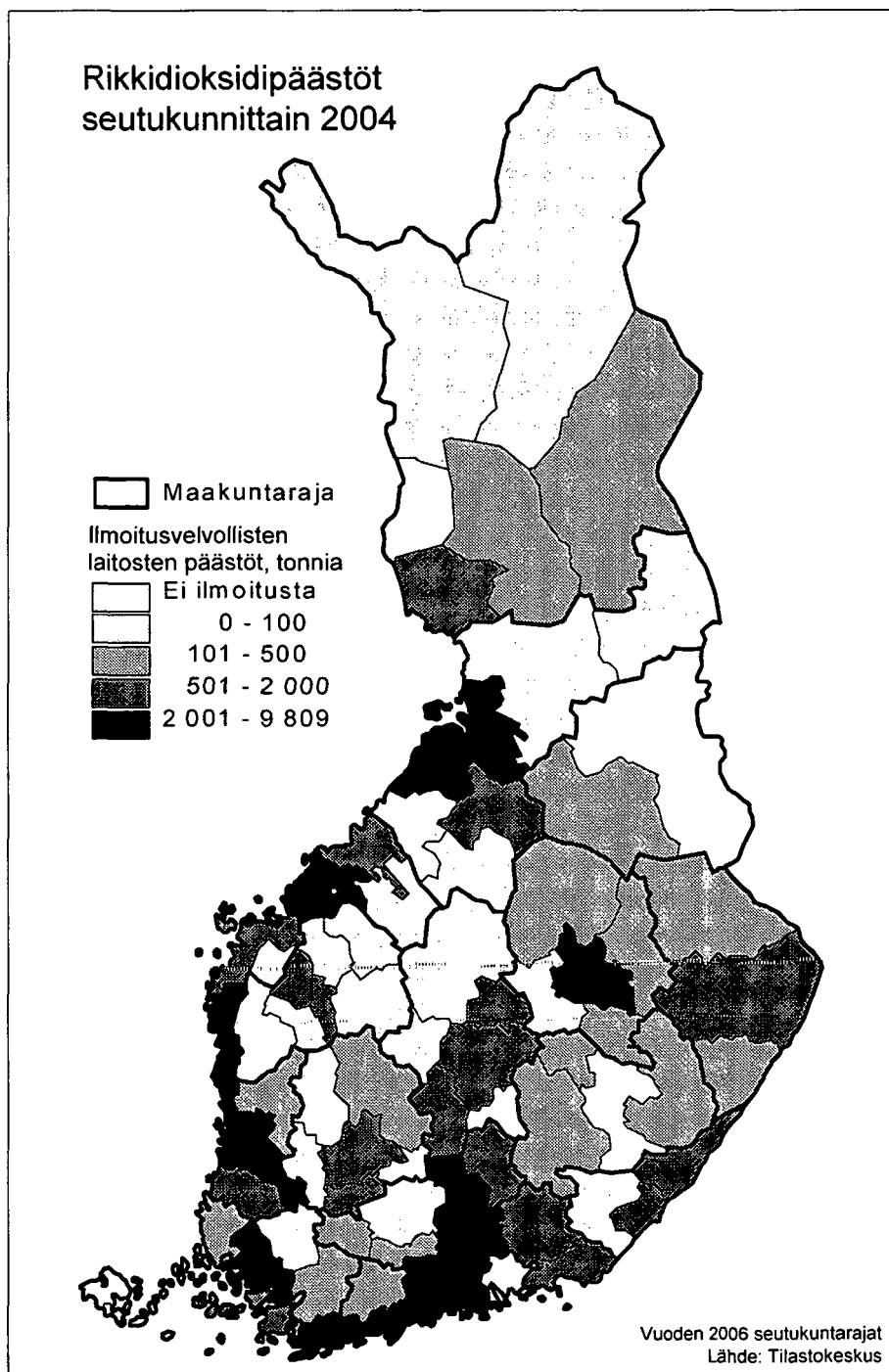
Kuva 18.6. Rikkidioksidipäästöt seutukunnittain 2004.
