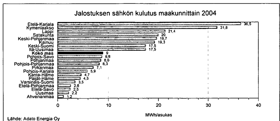
Kuva 4.6. Jalostuksen sähkön kulutus maakunnittain 2004.
