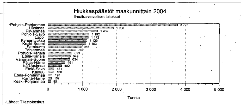
Kuva 18.5. Hiukkaspäästöt maakunnittain 2004.
