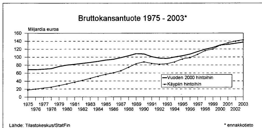
Kuva 5.1. Bruttokansantuote 1975–2003.
