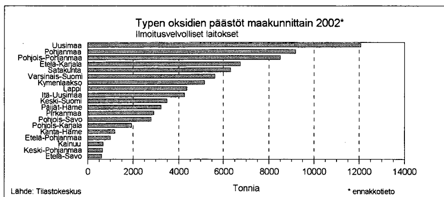
Kuva 12.2. Typen oksidien päästöt maakunnittain 2002.
