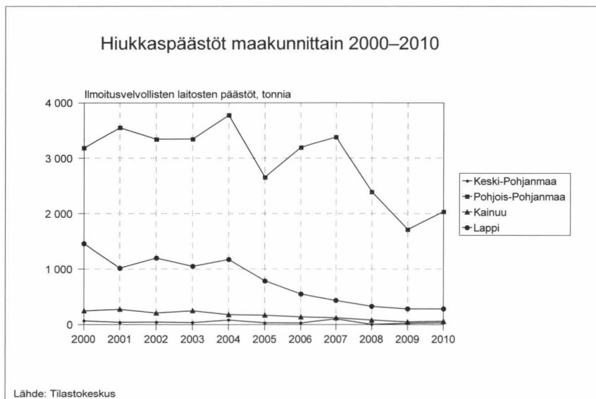
Kuva 13.5. Hiukkaspäästöt maakunnittain 2000–2010.
