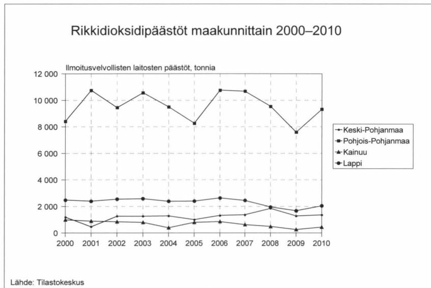
Kuva 13.4. Rikkidioksidipäästöt maakunnittain 2000–2010.
