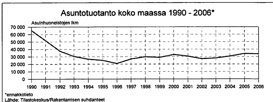
Kuva 12.3. Asuntotuotanto koko maassa 1990–2006.
