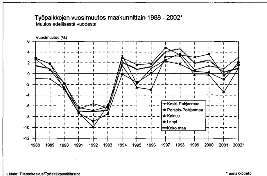
Kuva 6.5. Työpaikkojen vuosimuutos maakunnittain 1988 - 2002.
