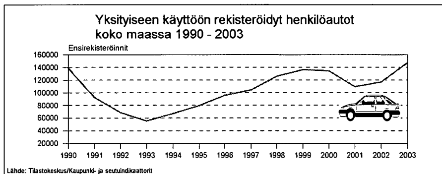
Kuva 10.1. Yksityiseen käyttöön rekisteröidyt henkilöautot koko maassa 1990 - 2003.
