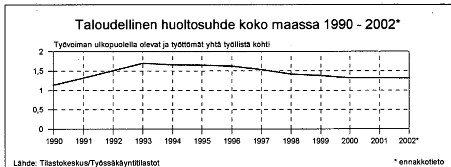
Kuva 6.1. Taloudellinen huoltosuhde koko maassa 1990 – 2002.
