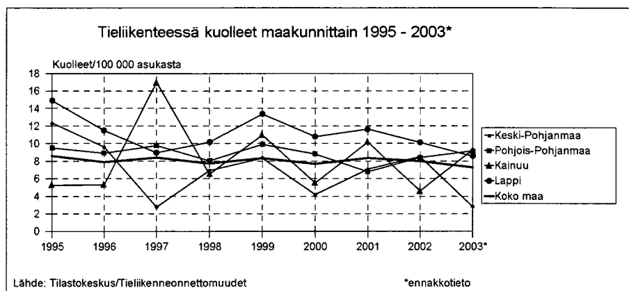
Kuva 10.4. Tieliikenteessä kuolleet maakunnittain 1995 - 2003.
