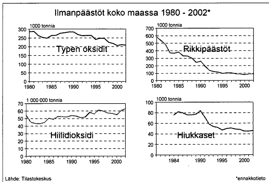
Kuva 12.1. Ilmanpäästöt koko maassa 1980 - 2002.
