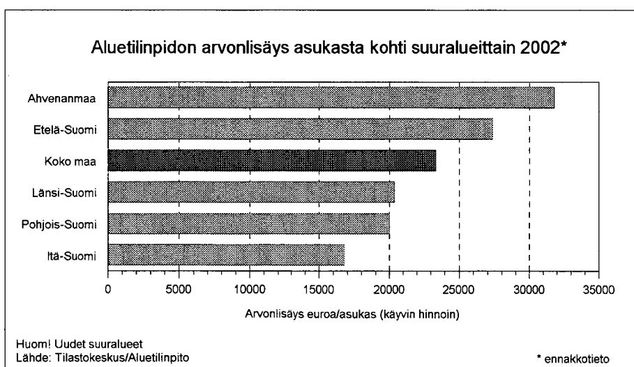
Kuva 5.2. Aluetilinpidon arvonlisäys asukasta kohti suuralueittain 2002.
