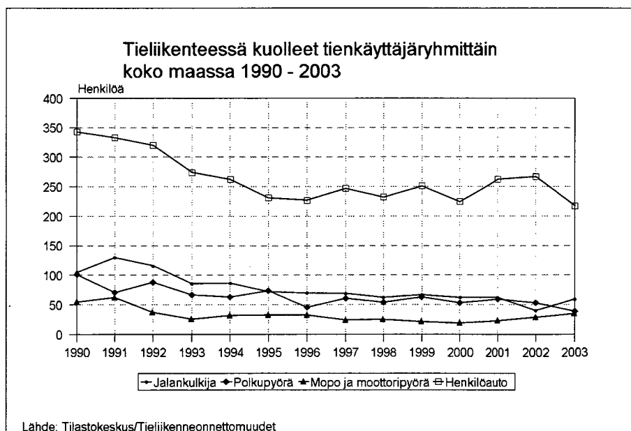
Kuva 10.5. Tieliikenteessä kuolleet tienkäyttäjärhmittäin koko maassa 1990 - 2003.
