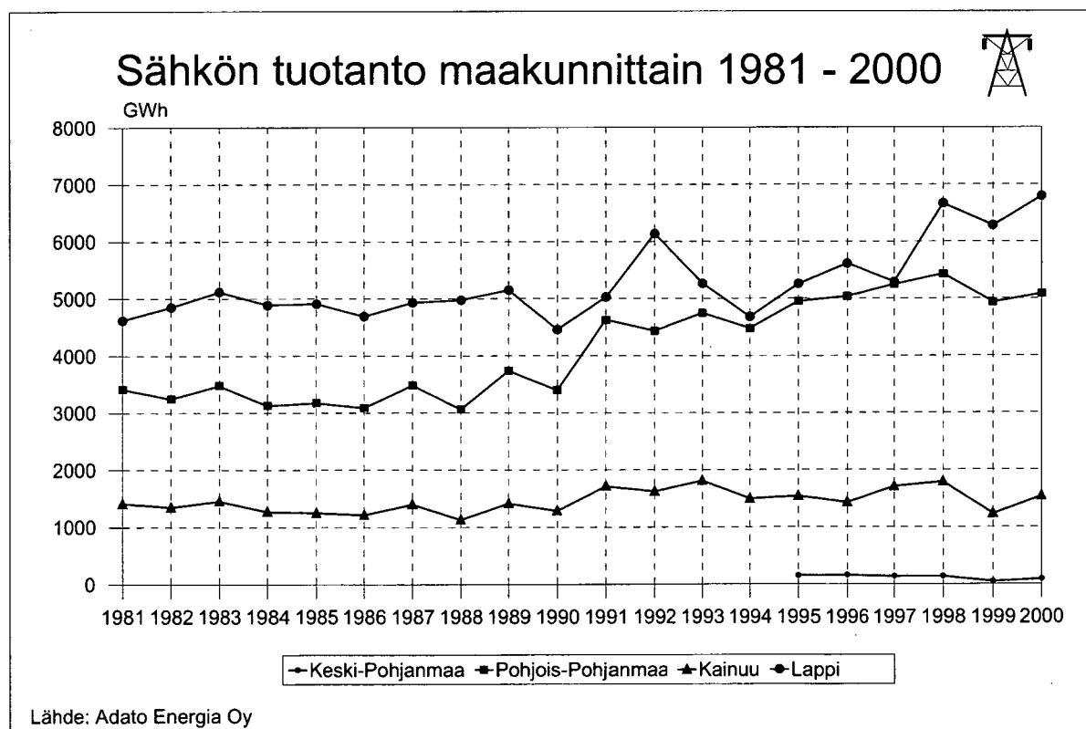
Kuva 118. Sähkön tuotanto maakunnittain 1981 – 2000.
