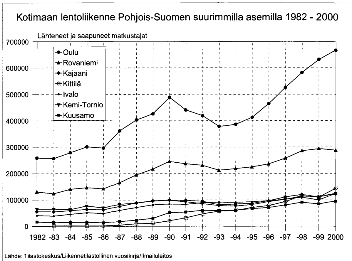
Kuva 111. Kotimaan lentoliikenne Pohjois-Suomen suurimmilla asemilla 1982 - 2000.
