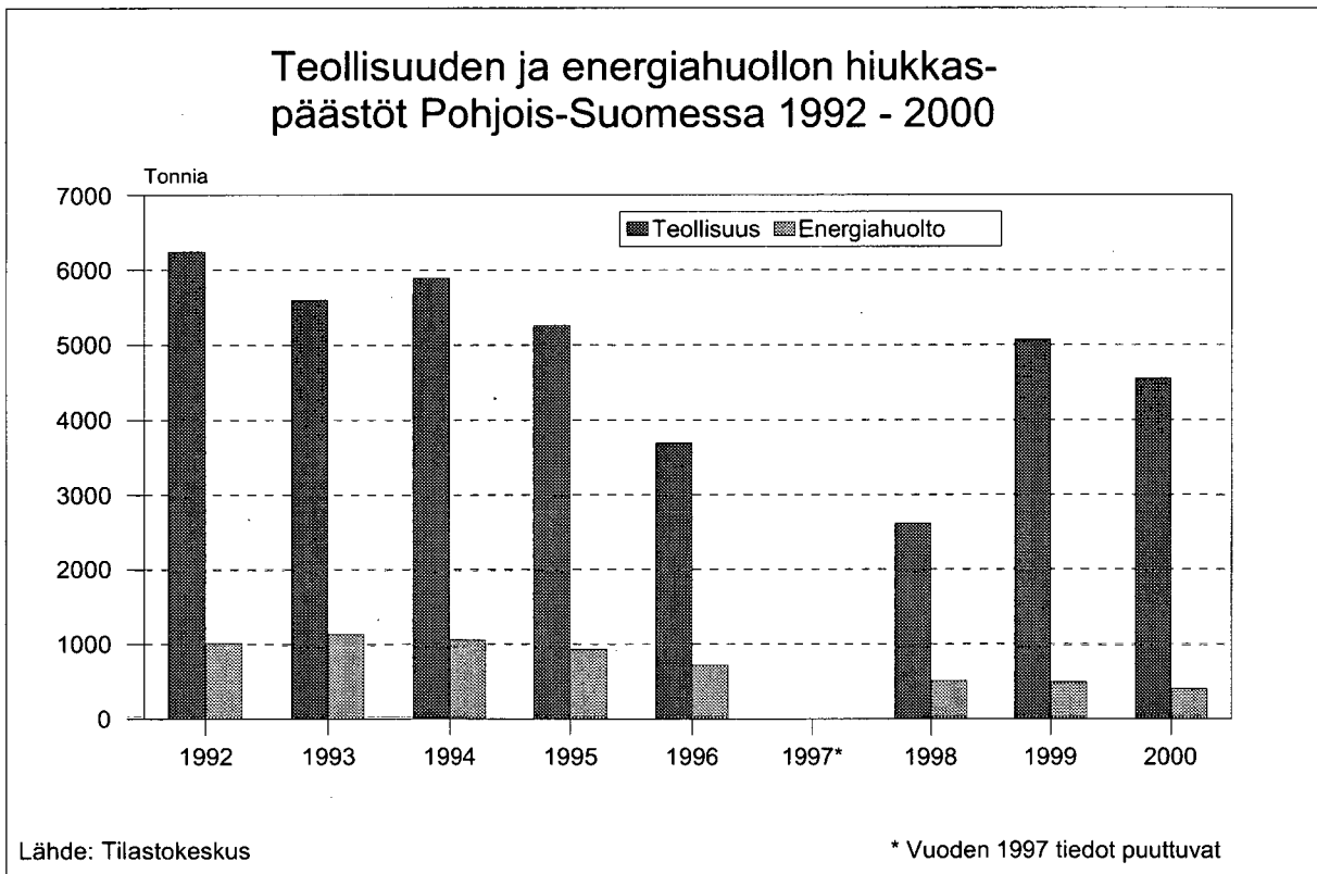
Kuva 127. Teollisuuden ja energiahuollon hiukaspäästöt Pohjois-Suomessa 1992 - 2000.
