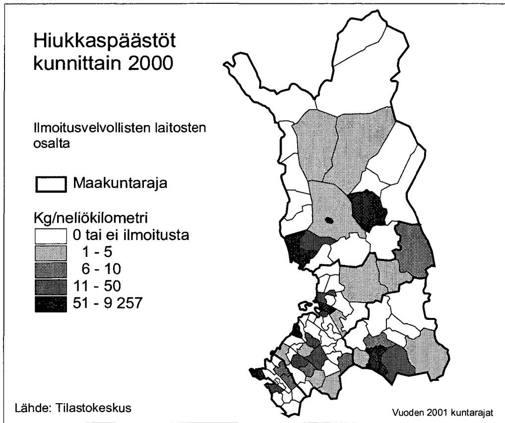
Kuva 130. Hiukkaspäästöt kunnittain 2000.
