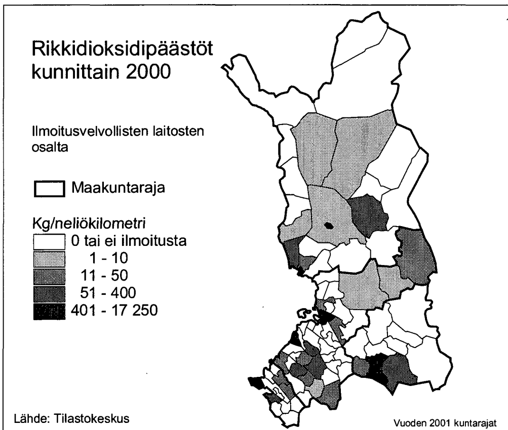
Kuva 129. Rikkidioksidipäästöt ( \text{SO}_2 ) kunnittain 2000.
