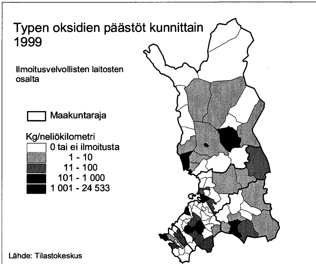
Kuva 123. Typen oksidien päästöt ( \text{No}_x ) kunnittain 1999.
