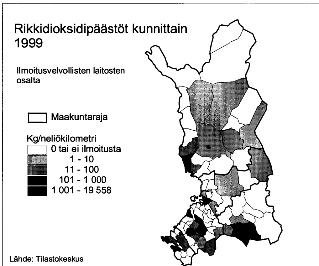
Kuva 124. Rikkidioksidipäästöt ( \text{SO}_2 ) kunnittain 1999.
