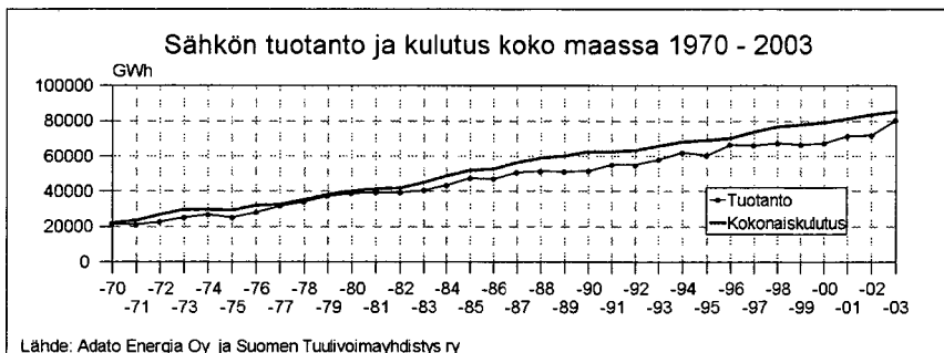
Kuva 4.1. Sähkön tuotanto ja kulutus koko maassa 1970–2003.
