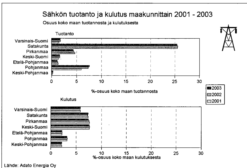
Kuva 4.2. Sähkön tuotanto ja kulutus maakunnittain 2001–2003.
