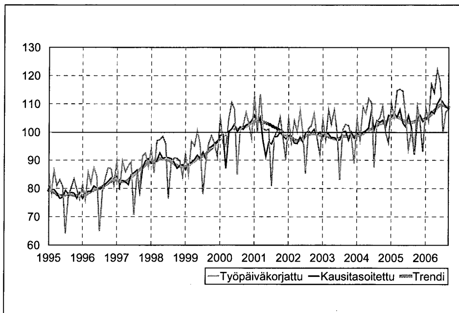
Kuvio 8. Kemianteollisuus TOL 23-25, teollisuustuotannon volyyymi-indeksi 1995 – 2006 syyskuu, 2000=100
