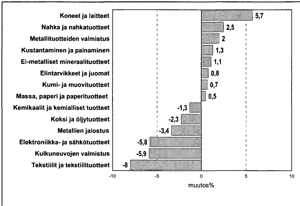
Kuvio 3. Teollisuustuotannon kausitasoitettu muutosprosentti elokuu 2004 / syyskuu 2004
