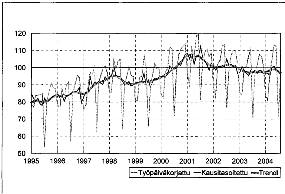
Kuvio 9. Muu metalliteollisuus TOL met - DL, teollisuustuotannon volyymi-indeksi 1995 – 2004 elokuu, 2000=100
