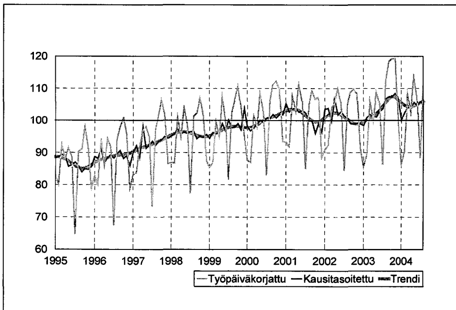
Kuvio 6. Muu tehdasteollisuus TOL 15, 17, 18, 19, 22, 26, 36, 37 teollisuustuotannon volyymi-indeksi 1995 – 2004 elokuu, 2000=100
