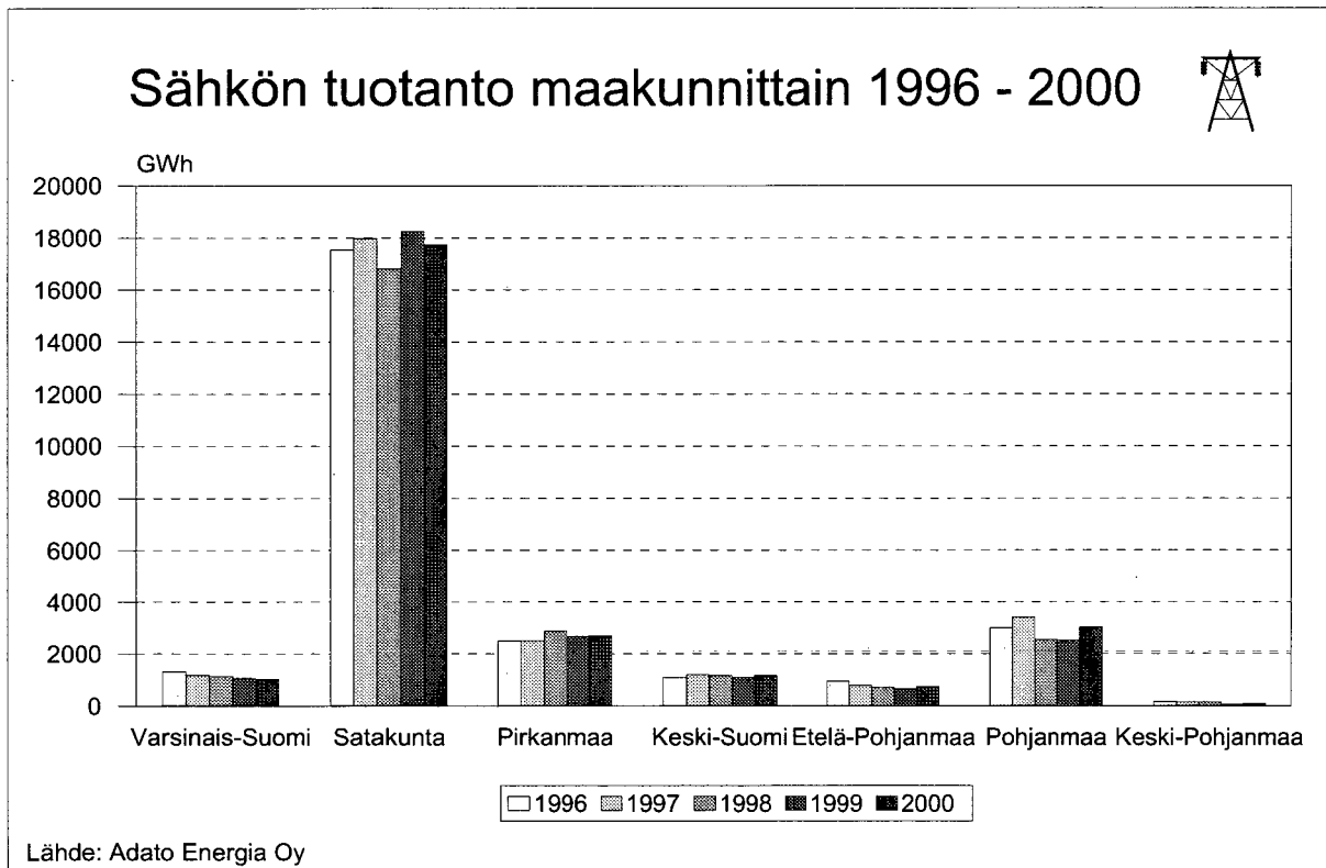
Kuva 108. Sähkön tuotanto maakunnittain 1996 – 2000.
