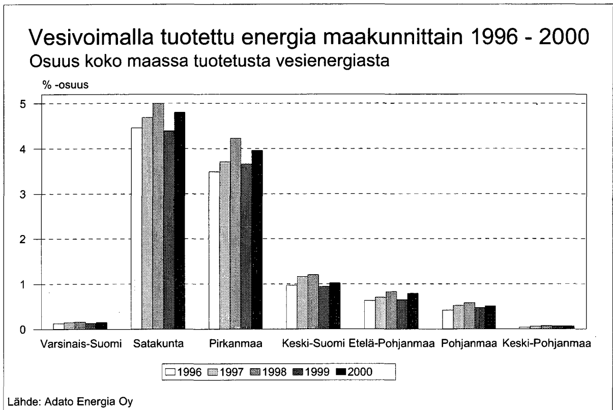
Kuva 113. Vesivoimalla tuotettu energia maakunnittain 1996 – 2000.
