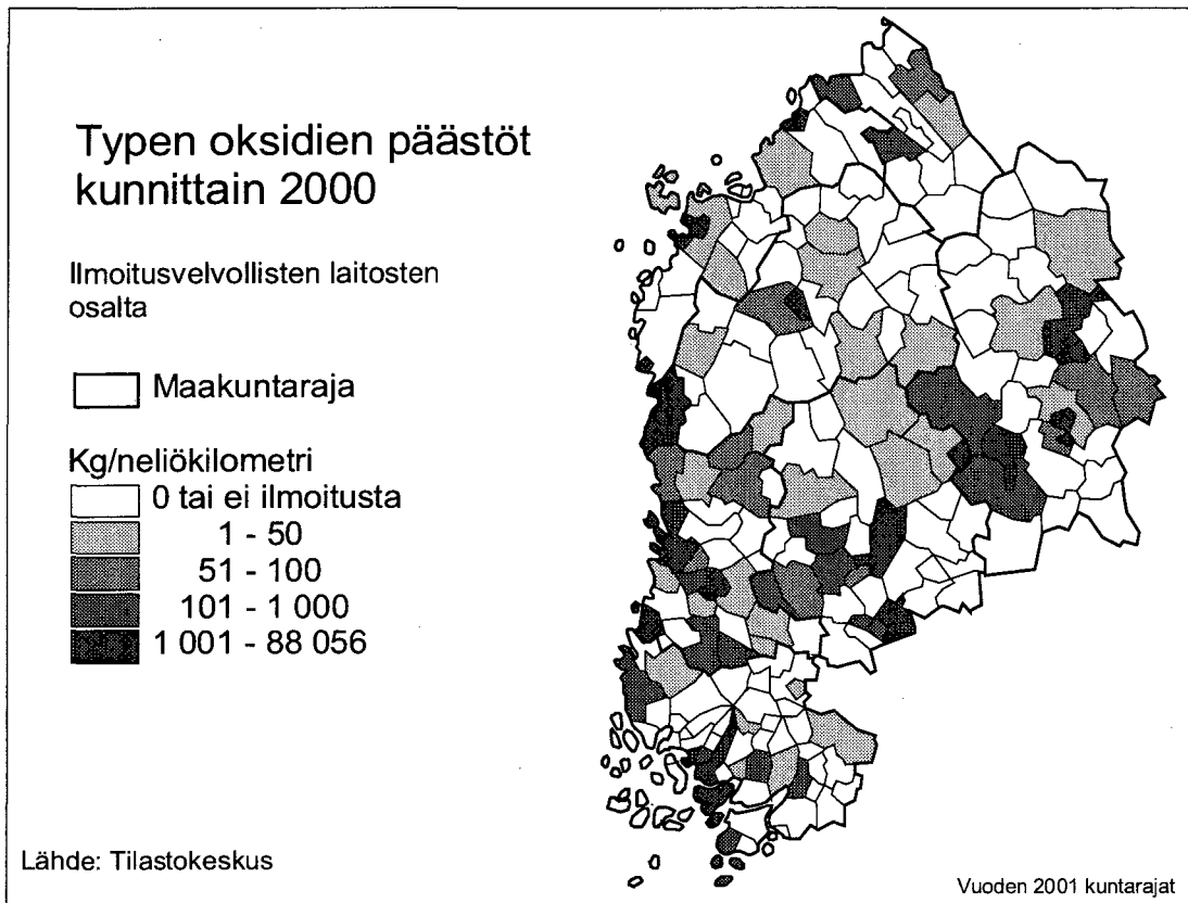
Kuva 118. Typen oksidien päästöt ( \text{No}_x ) kunnittain 2000.
