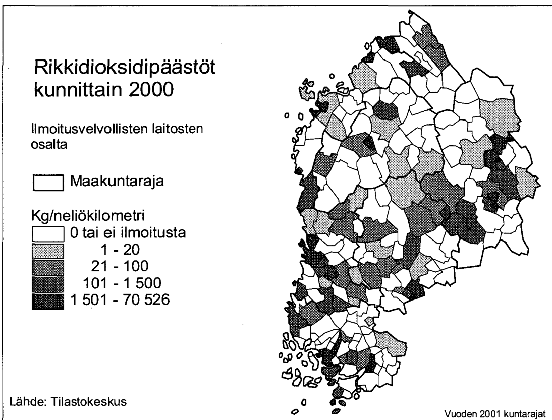
Kuva 119. Rikkidioksidipäästöt ( \text{SO}_2 ) kunnittain 2000.
