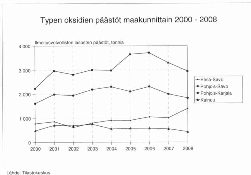
Kuva 15.3. Typen oksidien päästöt maakunnittain 2000–2008.
