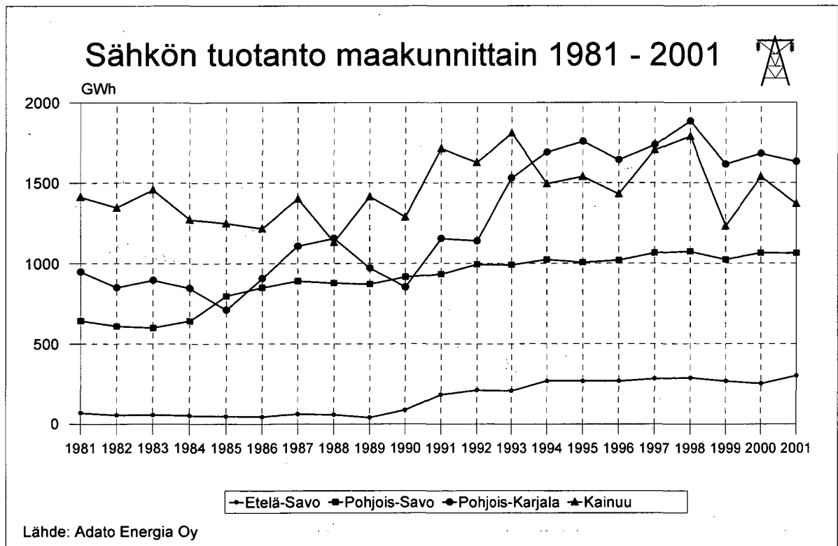
Kuva 135. Sähkön tuotanto maakunnittain 1981–2001.
