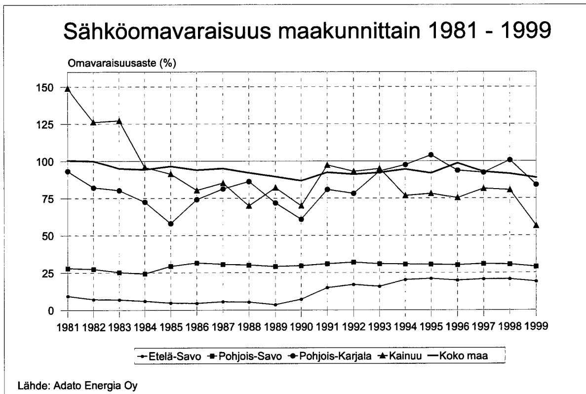
Kuva 119. Sähköomavaraisuus maakunnittain 1981 – 1999.
