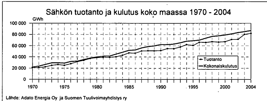
Kuva 4.1. Sähkön tuotanto ja kulutus koko maassa 1970–2004.
