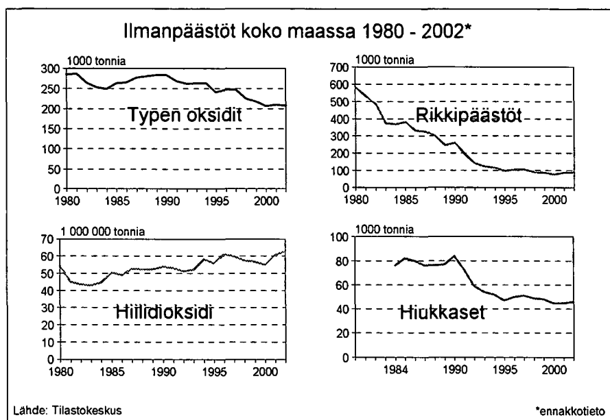
Kuva 12.1. Ilmanpäästöt koko maassa 1980–2002.
