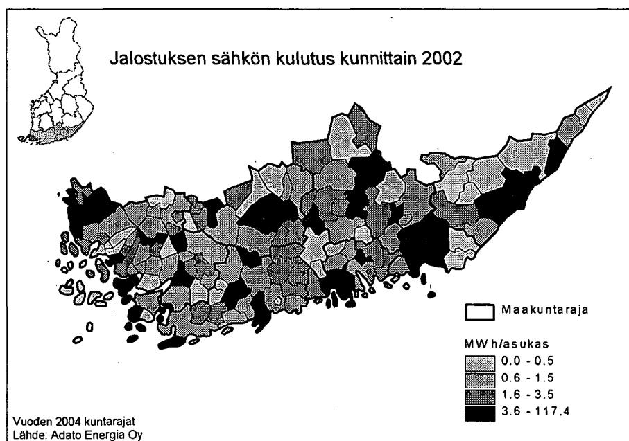
Kuva 11.3. Jalostuksen sähkön kulutus kunnittain 2002.
