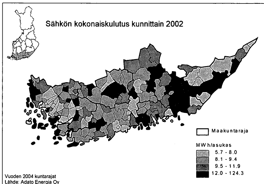
Kuva 11.6. Sähkön kokonaiskulutus kunnittain 2002.
