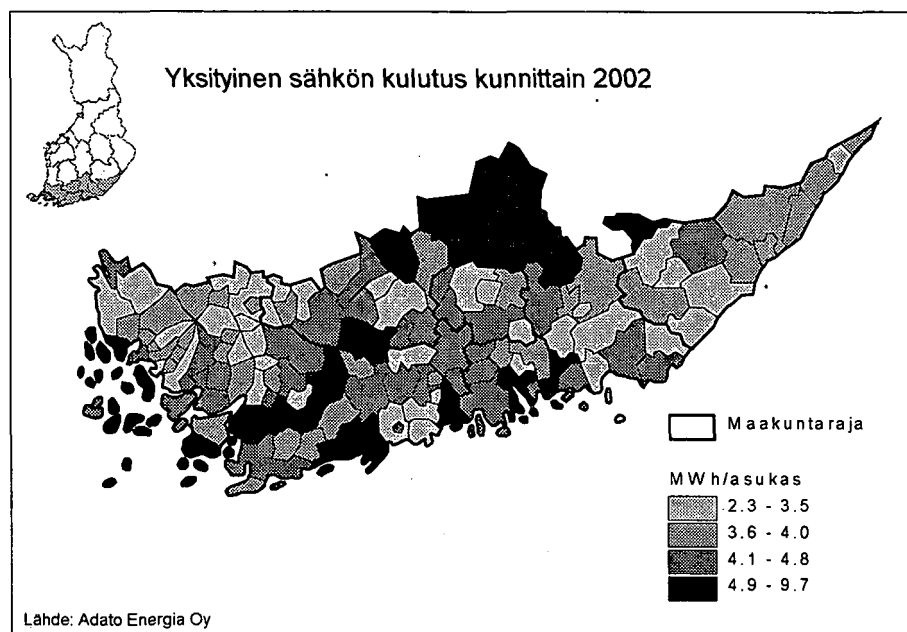
Kuva 11.4. Yksityinen sähkön kulutus kunnittain 2002.
