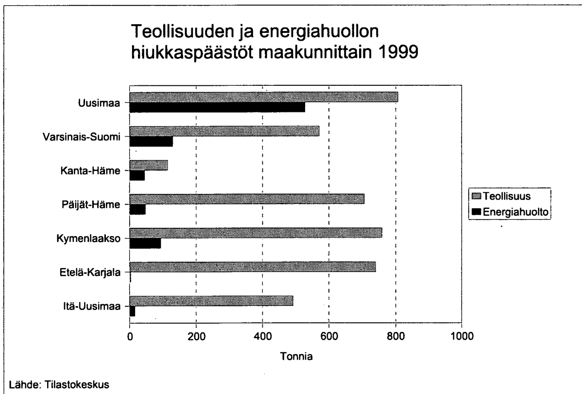
Kuva 115. Teollisuuden ja energiahuollon hiukkaspäästöt maakunnittain 1999.
