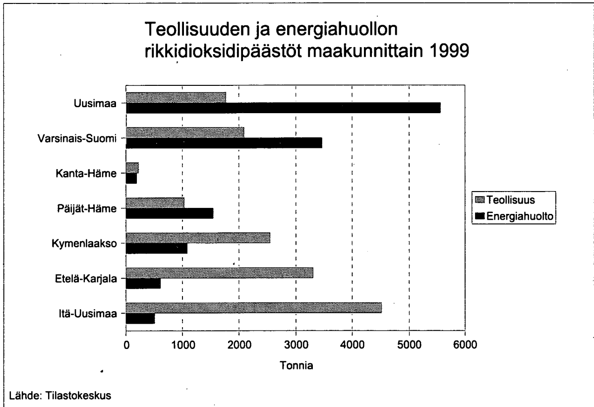
Kuva 114. Teollisuuden ja energiahuollon rikkidioksidipäästöt maakunnittain 1999.
