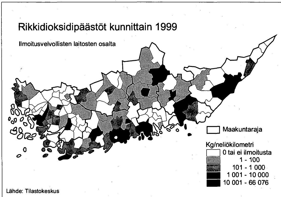
Kuva 117. Rikkidioksidipäästöt ( \text{SO}_2 ) kunnittain 1999.
