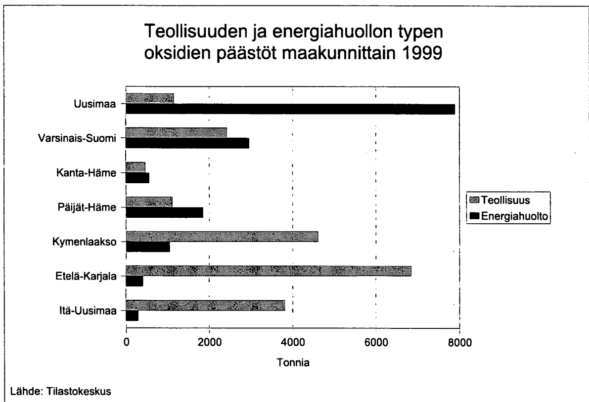
Kuva 113. Teollisuuden ja energiahuollon typen oksidien päästöt maakunnittain 1999.
