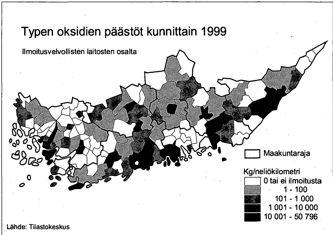
Kuva 116. Typen oksidien päästöt ( \text{No}_x ) kunnittain 1999.
