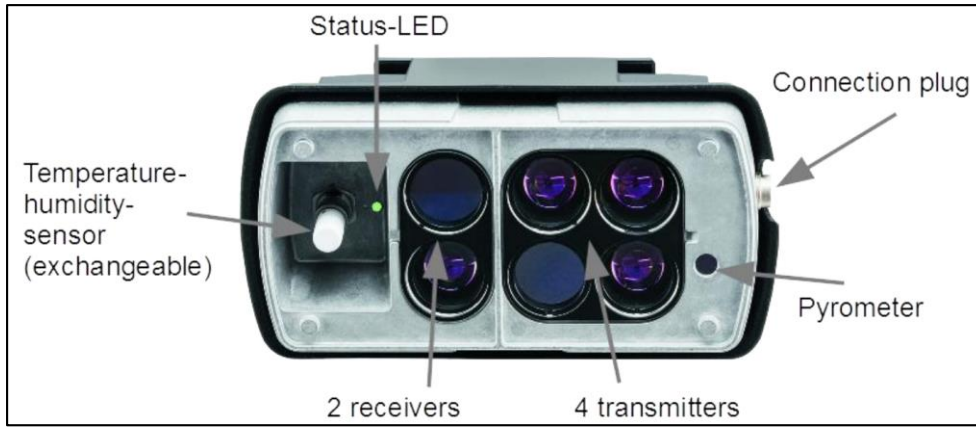
Kuva 4. STARWIS/MARWIS-sensori (Lufft, 2017).
