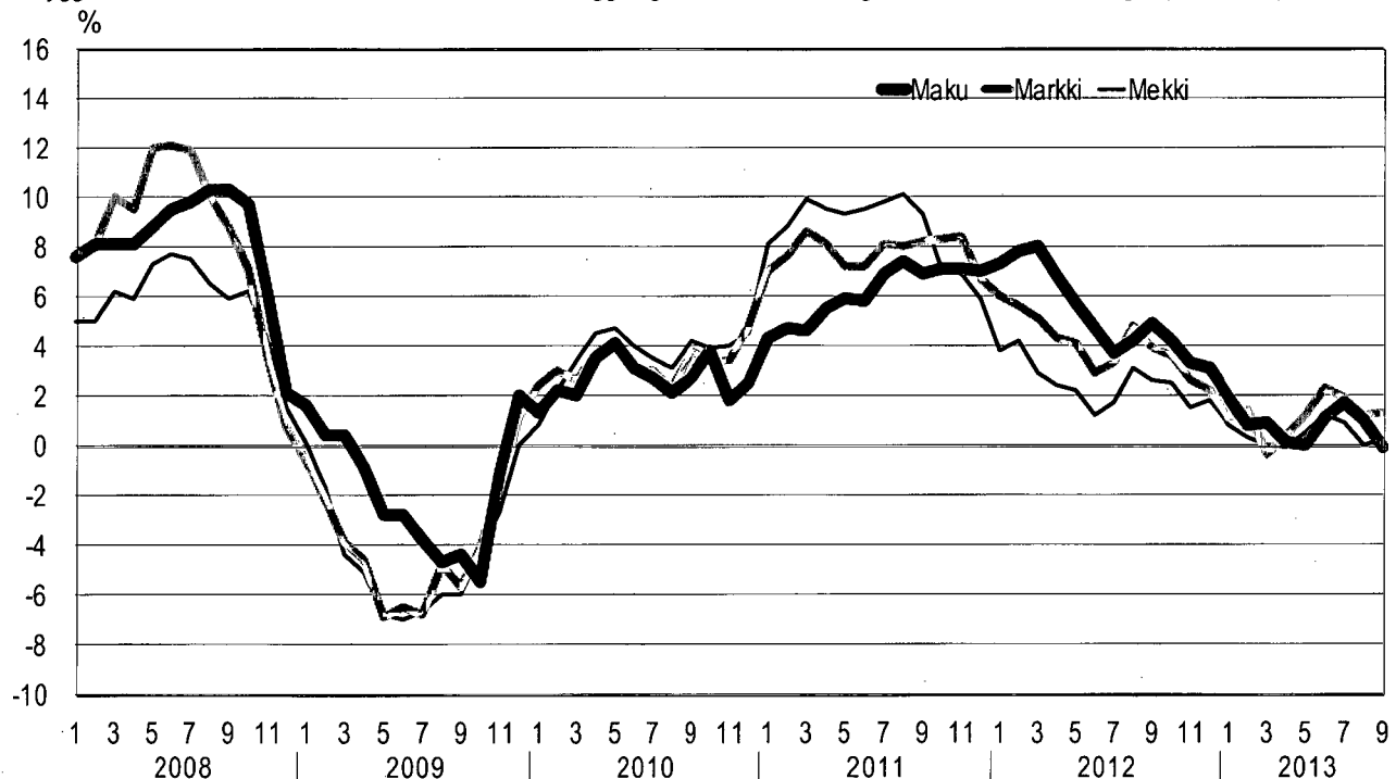
Maarakennuskustannusindeksin sekä maarakennusalan ja metsäalan konekustannusindeksien vuosimuutokset (2005=100) Jordbyggnadskostnadsindex samt kostnadsindex för anläggningsmaskiner och skogsmaskiner, årsförändringar (2005=100)
