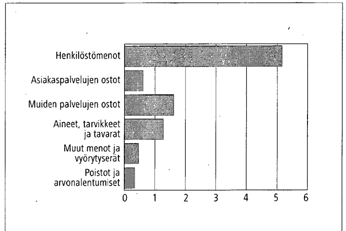
Kuvio 5. Käyttökustannukset (mrd. euroa) menolajeittain 2008
