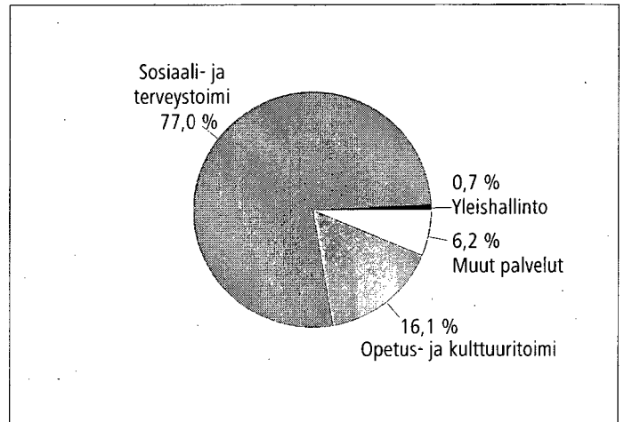
Kuvio 4. Käyttökustannukset tehtävittäin, %, 2008
