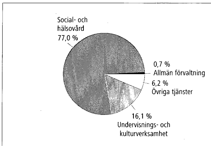
Figur 4. Driftskostnader efter uppgift, %, 2008
