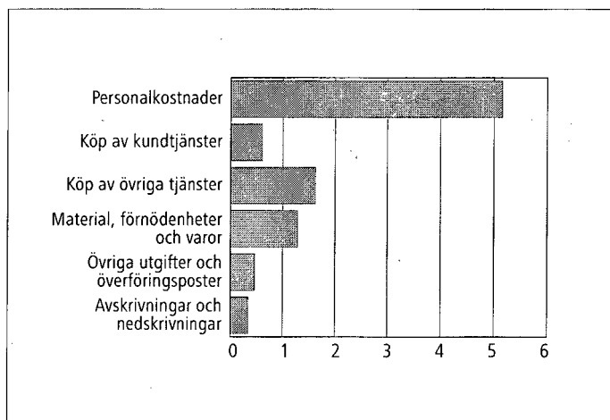
Figur 5. Driftskostnader (mrd. euro) efter utgiftslag 2008
