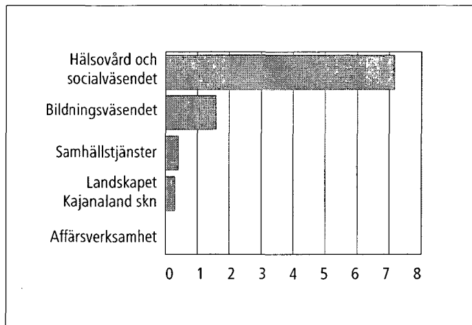
Figur 1. Driftskostnader (mrd.euro) efter samkommunstyp 2008
