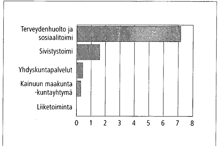
Kuvio 1. Käyttökustannukset (mrd. euroa) kuntayhtymätyypeittäin vuonna 2008
