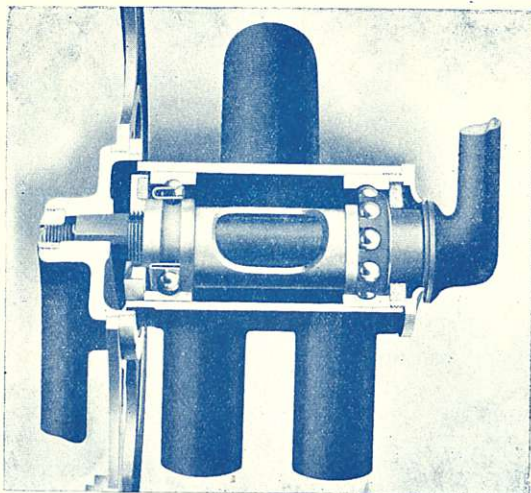
Keskuosa kuularengaslaakerilla ja itsetoimivalla voitelulaitteella.
